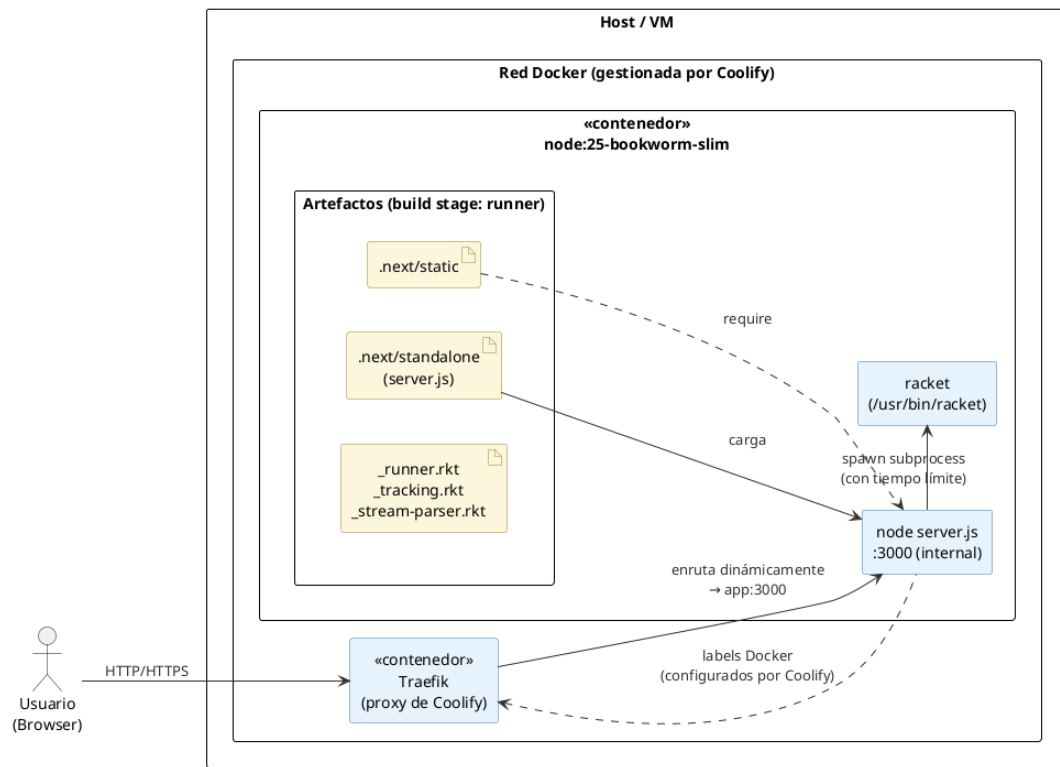
Figura 5.8: Diagrama de despliegue del prototipo FLP Viewer en el entorno de pruebas
