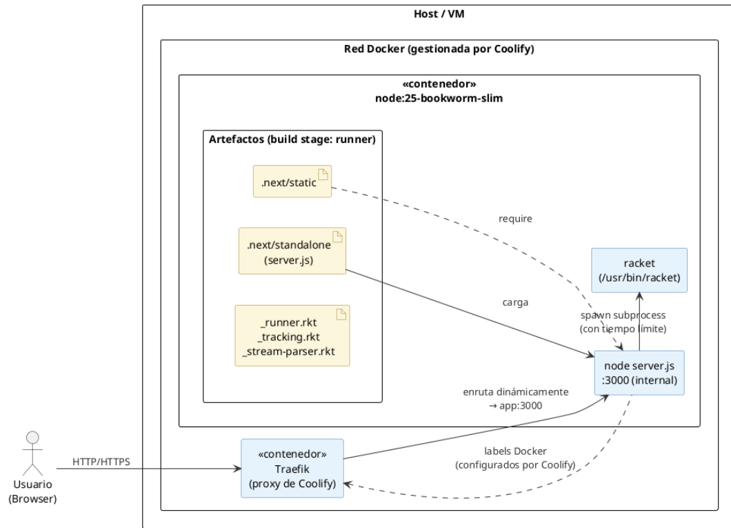
Figura 5.8: Diagrama de despliegue del prototipo FLP Viewer en el entorno de pruebas
