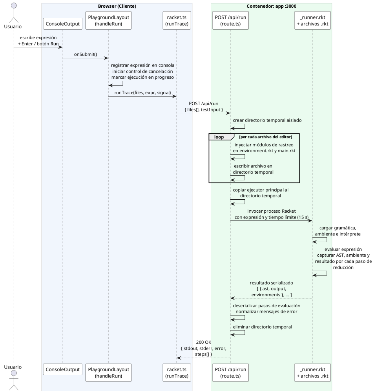
Figura 5.6: Diagrama de secuencia de la solicitud y evaluación en el servidor del prototipo FLP Viewer
