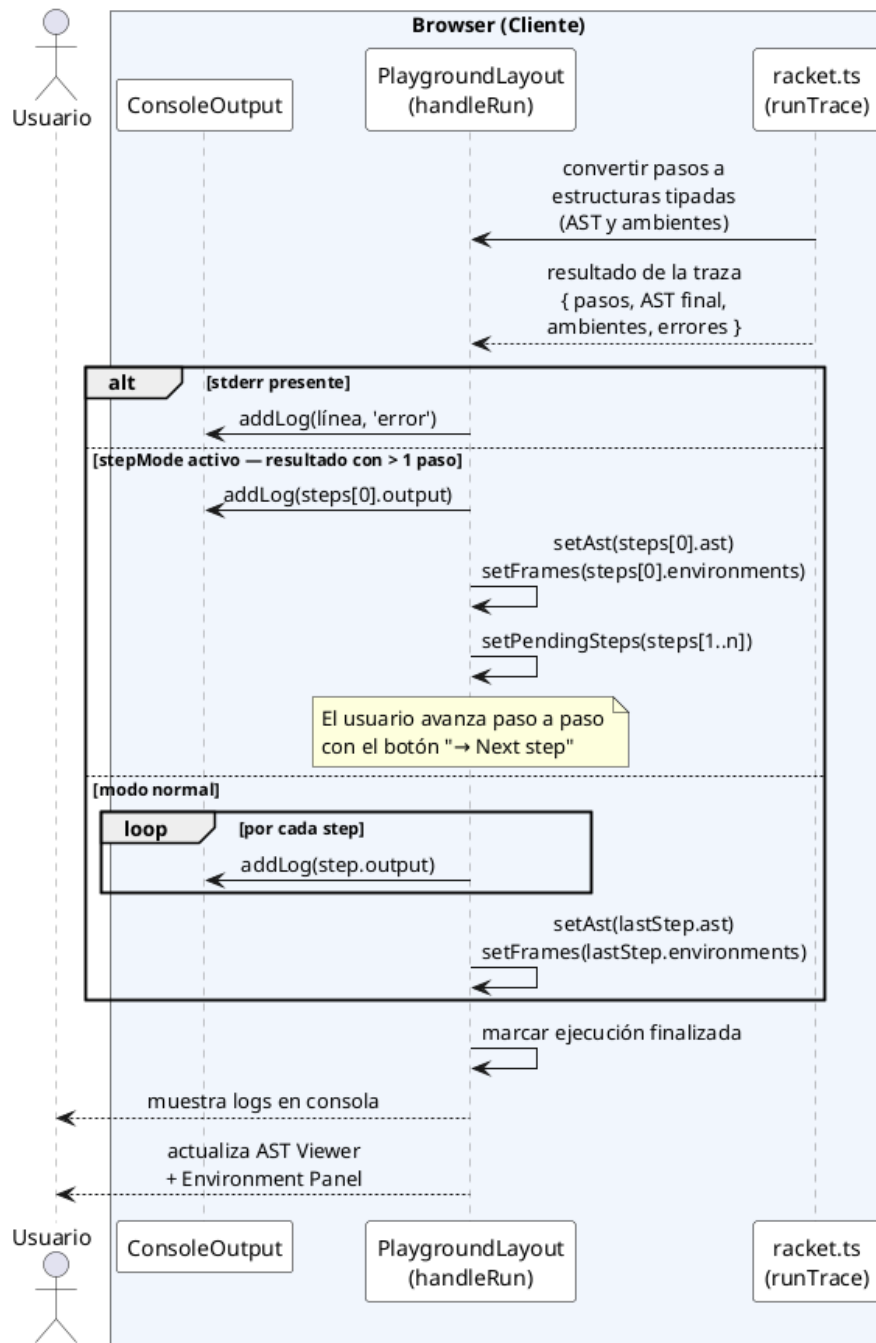
Figura 5.7: Diagrama de secuencia de la distribución de resultados en la interfaz del prototipo FLP Viewer
