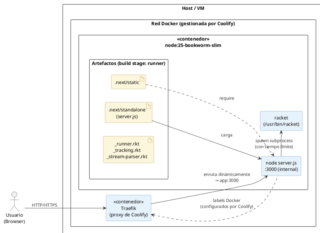
Figura 5.8: Diagrama de despliegue del prototipo FLP Viewer en el entorno de pruebas Fuente: Elaboración propia
