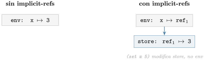
Figura 2.3: Comparación entre el modelo sin IMPLICIT-REFS, donde el ambiente almacena directamente el valor, y el modelo con IMPLICIT-REFS, donde el ambiente almacena una referencia hacia una celda mutable en el store .
