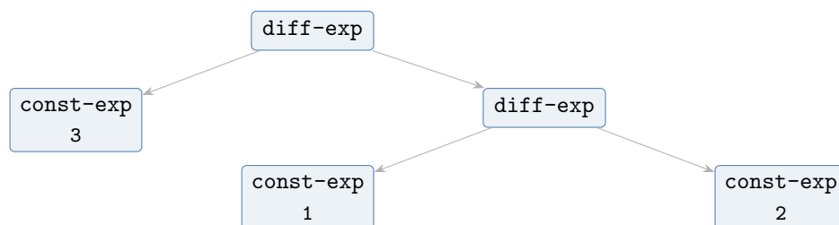
Figura 2.1: AST de (diff 3 (diff 1 2)) : cada producción BNF origina un constructor del tipo de datos.
