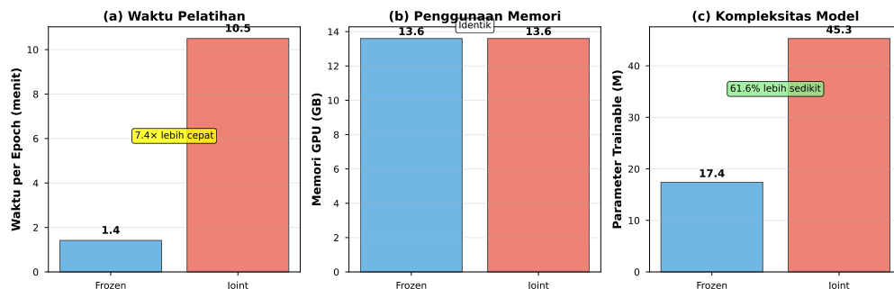
Gambar V.8 Efisiensi komputasi: (a) Frozen 7.4\times lebih cepat (85s vs 630s per epoch). (b) Memori identik (13.6 GB). (c) Pengurangan parameter trainable 61.6% (17.4M vs 45.3M) berkontribusi pada kecepatan DAN stabilitas.
