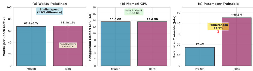
Gambar 6: Perbandingan efisiensi komputasi antara frozen recognizer dan joint training . (a) Waktu pelatihan per epoch : frozen 67.4 ± 0.7 detik ( frozen : training only, joint : training + validasi), joint 68.1 ± 1.5 detik (dari analisis timestamp ). (b) Penggunaan memori GPU: hampir identik (~13.6 GB), pembekuan recognizer tidak memberikan keuntungan memori signifikan. (c) Jumlah parameter trainable : frozen 61.6% lebih sedikit (17.4M vs ~45.3M), berkontribusi pada stabilitas pelatihan dan pencegahan kelupaan katastropik .
