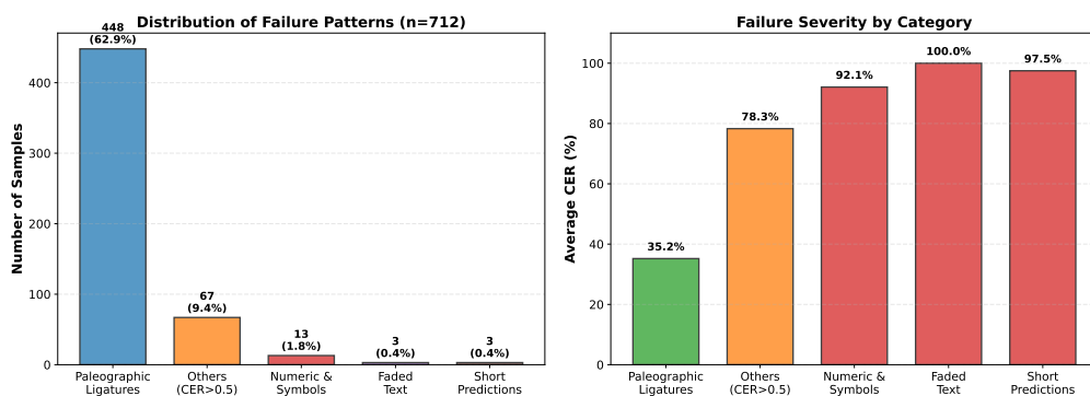
Gambar V.18 Distribusi pola kegagalan (kiri) dan tingkat keparahan CER (kanan) pada set uji ( n=712 ). Ligatur paleografi mendominasi (62.9% dari kasus CER tinggi) dengan CER moderat (35.2%), sementara kasus jarang seperti teks memudar ekstrem dan artefak simbol menunjukkan kegagalan parah (CER \approx 100%). Hasil ini mengindikasikan bahwa mayoritas kesalahan bersumber dari kompleksitas intrinsik tulisan tangan paleografi abad ke-16 hingga ke-18, bukan dari kegagalan restorasi total.
