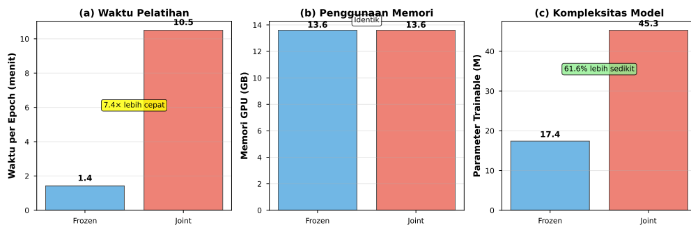
Gambar V.8 Efisiensi komputasi: (a) Frozen 7.4\times lebih cepat (85s vs 630s per epoch). (b) Memori identik (13.6 GB). (c) Pengurangan parameter trainable 61.6% (17.4M vs 45.3M) berkontribusi pada kecepatan DAN stabilitas.
