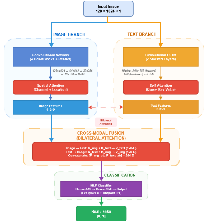
Fig. 4: Arsitektur Diskriminator Dual-Modal Enhanced dengan bilateral cross-modal attention: cabang CNN (512-D) dengan spatial attention, cabang BiLSTM (512-D) dengan self-attention. Fusion bilateral (128-D) untuk validasi holistik.
