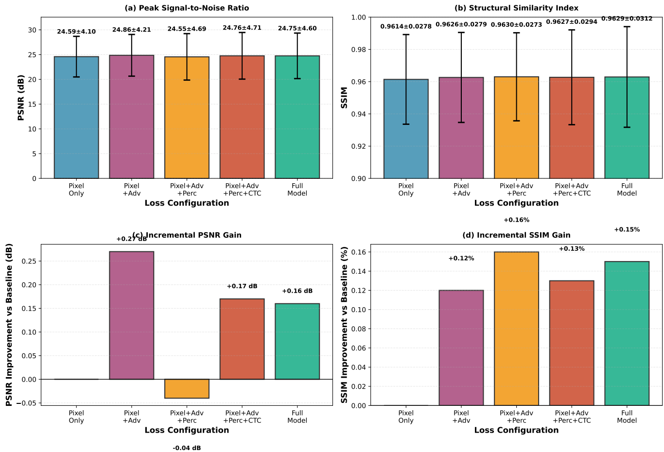
Fig. 11: Studi ablati inkremental komponen loss: (a–b) Metrik absolut PSNR dan SSIM untuk setiap konfigurasi, (c–d) Peningkatan inkremental relatif terhadap baseline hanya-piksel. Error bars menunjukkan deviasi standar pada validation set. Loss adversarial memberikan peningkatan PSNR tertinggi (+0.27 dB), sementara loss perseptual mengoptimalkan kesamaan struktural (+0.0016 SSIM).
