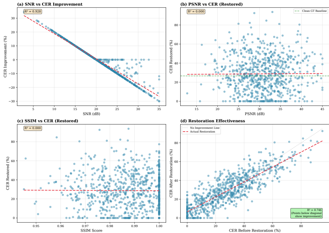
Gambar 13: Analisis korelasi tingkat degradasi pada set validasi (n=710): (a) korelasi negatif kuat (Pearson r=-0,963 , p<0,001 ) antara SNR dan peningkatan CER menunjukkan restorasi lebih efektif pada dokumen sangat terdegradasi, (b) PSNR vs CER pascarestorasi menunjukkan model membawa semua tingkat degradasi mendekati nilai referensi citra bersih (26,6%, garis hijau), (c) SSIM vs CER menunjukkan korelasi lemah mengindikasikan kesamaan struktural bukan prediktor tunggal untuk akurasi HTR, (d) perbandingan CER sebelum-sesudah menunjukkan mayoritas sampel mengalami perbaikan (poin di bawah diagonal y=x , abu-abu). Catatan: Data dari set validasi (n=710) dengan statistik PSNR 30,91\pm5,60 dB, CER 27,11\pm20,83\% , SSIM 0,987\pm0,014 . Hasil akhir pada set uji (n=712) dilaporkan dalam Tabel ??: PSNR 30.74 dB, CER 34.9%, SSIM 0.987.
