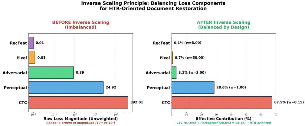
Gambar 11: Mekanisme inverse scaling yang muncul dari tuning manual bobot komponen loss . Panel kiri menunjukkan magnitude raw dengan ketidakseimbangan 4 orders of magnitude ( 10^{-2} hingga 10^2 ). Panel kanan menampilkan kontribusi efektif setelah penerapan bobot manual yang secara retrospektif mengikuti pola inverse scaling , mencapai keseimbangan by design dengan dominasi CTC (67.5%) dan Perceptual (28.6%) untuk prioritas HTR.
