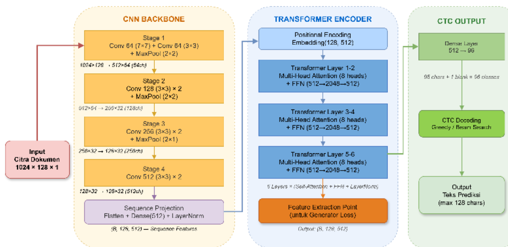
Gambar IV.4 Arsitektur HTR Recognizer : model hibrida CNN-Transformer dengan CNN Backbone 4 tahap (64 \rightarrow 512 kanal), Transformer Encoder 6 lapisan (8 heads, dimensi 512), dan CTC Output Layer (96 kelas). Total 27,86M parameter dibekukan selama pelatihan GAN.
