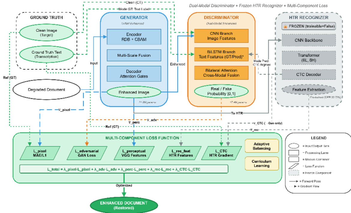
Gambar IV.1 Metode GAN-HTR dengan diskriminator dual-modal dan frozen HTR recognizer. Komponen utama: (1) Generator U-Net Enhanced , (2) Diskriminator Dual-Modal (CNN+BiLSTM), (3) Frozen HTR Recognizer untuk CTC loss.
