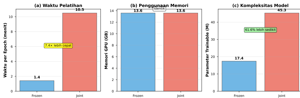
Gambar V.10 Analisis efisiensi: (a) waktu per epoch , (b) penggunaan memori GPU, (c) jumlah parameter dapat dilatih. Strategi frozen mengurangi beban komputasi 7,4× tanpa mengorbankan akurasi.
