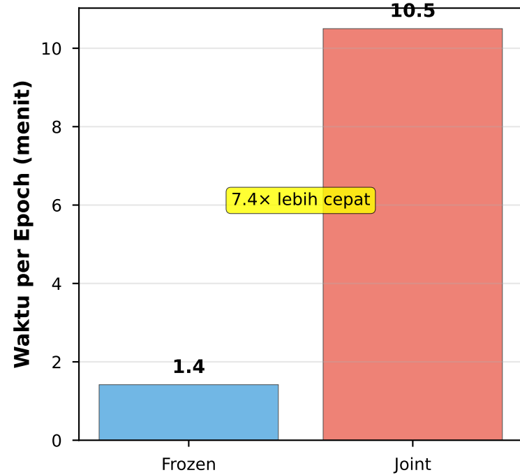
(a) Waktu Pelatihan
