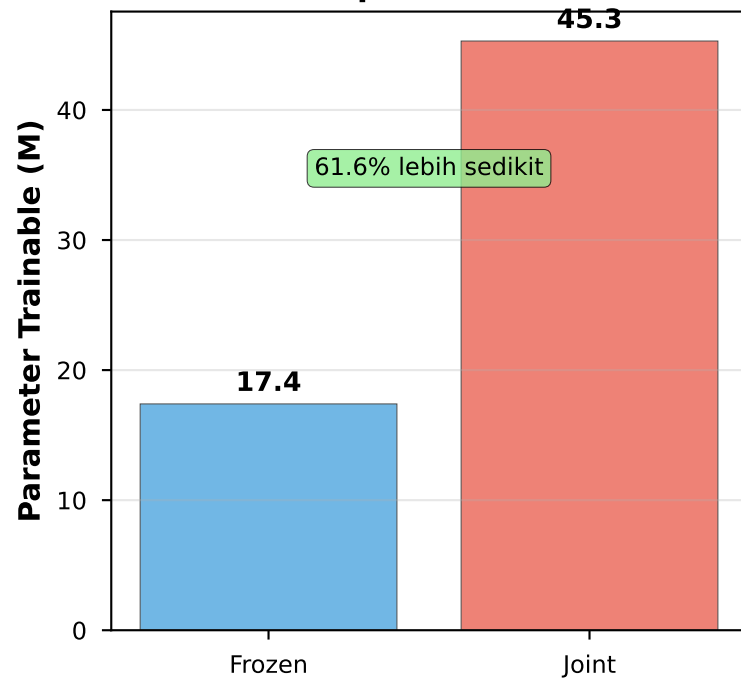
(c) Kompleksitas Model
