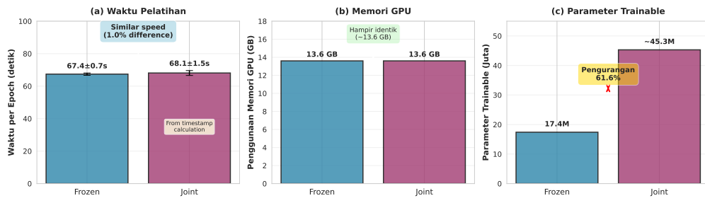
Gambar V.6 Perbandingan efisiensi komputasi antara frozen recognizer dan joint training . (a) Waktu pelatihan per epoch : frozen 67.4 ± 0.7 detik ( frozen : training only, joint : training + validasi), joint 68.1 ± 1.5 detik (dari analisis timestamp ). (b) Penggunaan memori GPU: hampir identik (~13.6 GB), pembekuan recognizer tidak memberikan keuntungan memori signifikan. (c) Jumlah parameter trainable : frozen 61.6% lebih sedikit (17.4M vs ~45.3M), berkontribusi pada stabilitas pelatihan dan pencegahan kelupaan katastropik .
