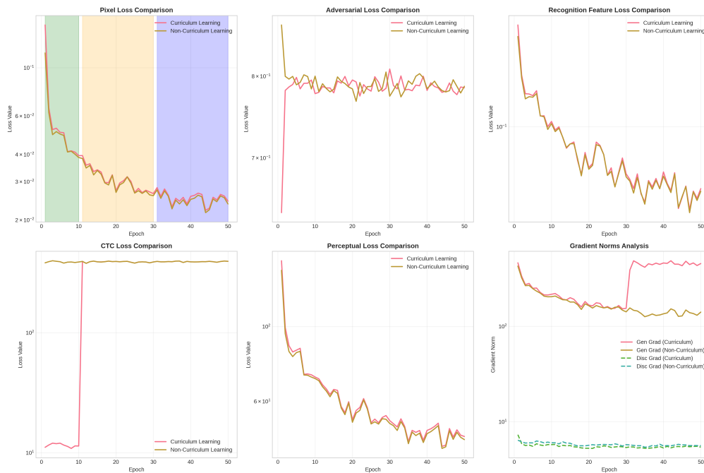
Gambar V.8 Analisis mendalam komponen loss: perbandingan evolusi pixel loss, adversarial loss, recognition feature loss, CTC loss, dan perceptual loss antara curriculum learning vs non-curriculum learning. Garis hijau menunjukkan fase warmup, orange menunjukkan fase transisi, dan biru menunjukkan fase pelatihan penuh.
