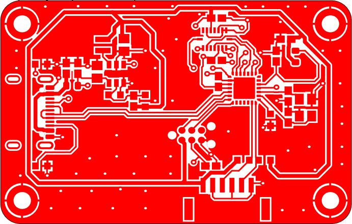
Top Layer (Scale 2:1)
