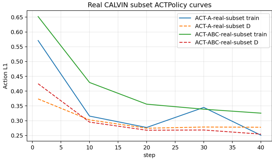
图 7: 真实 CALVIN 子集 ACTPolicy 的 Action L1 曲线。实线为训练 loss, 虚线为 D 子集评估 loss。
