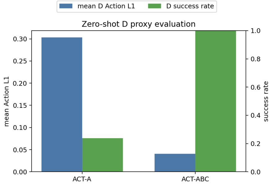
图 10: D 域 zero-shot 替代评估对比。
