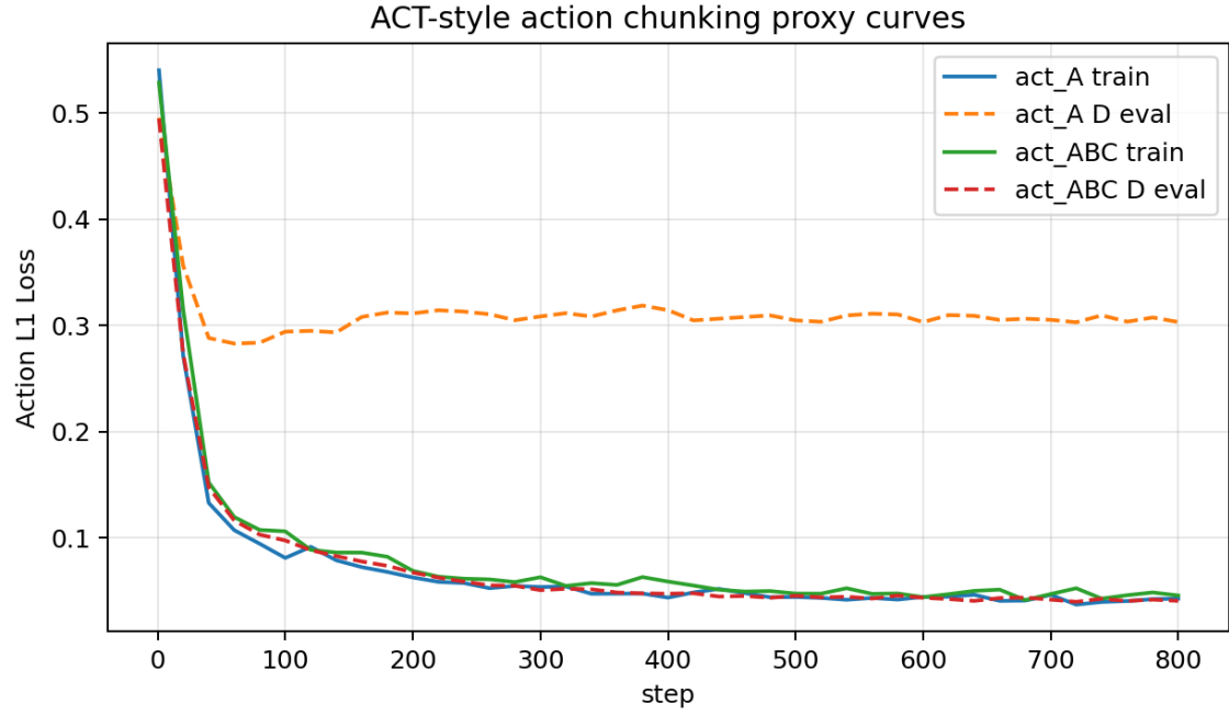
图 9: ACT 动作分块替代实验的 Action L1 曲线。实线为训练集 loss，虚线为 D 域评估 loss。
