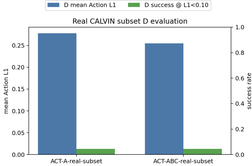
图 8: 真实 CALVIN 子集 D 域离线评估对比。
