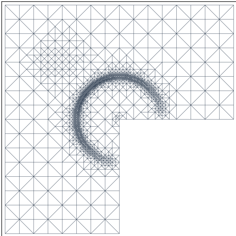
E2 AFEM final mesh (H-step 60) 3788 cells
