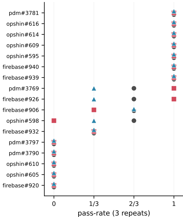
Codex (gpt-5.5)
