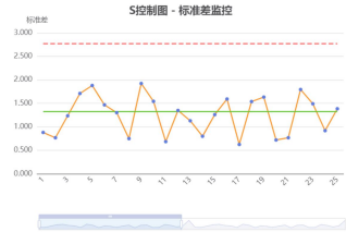
S控制图 (标准差图)
