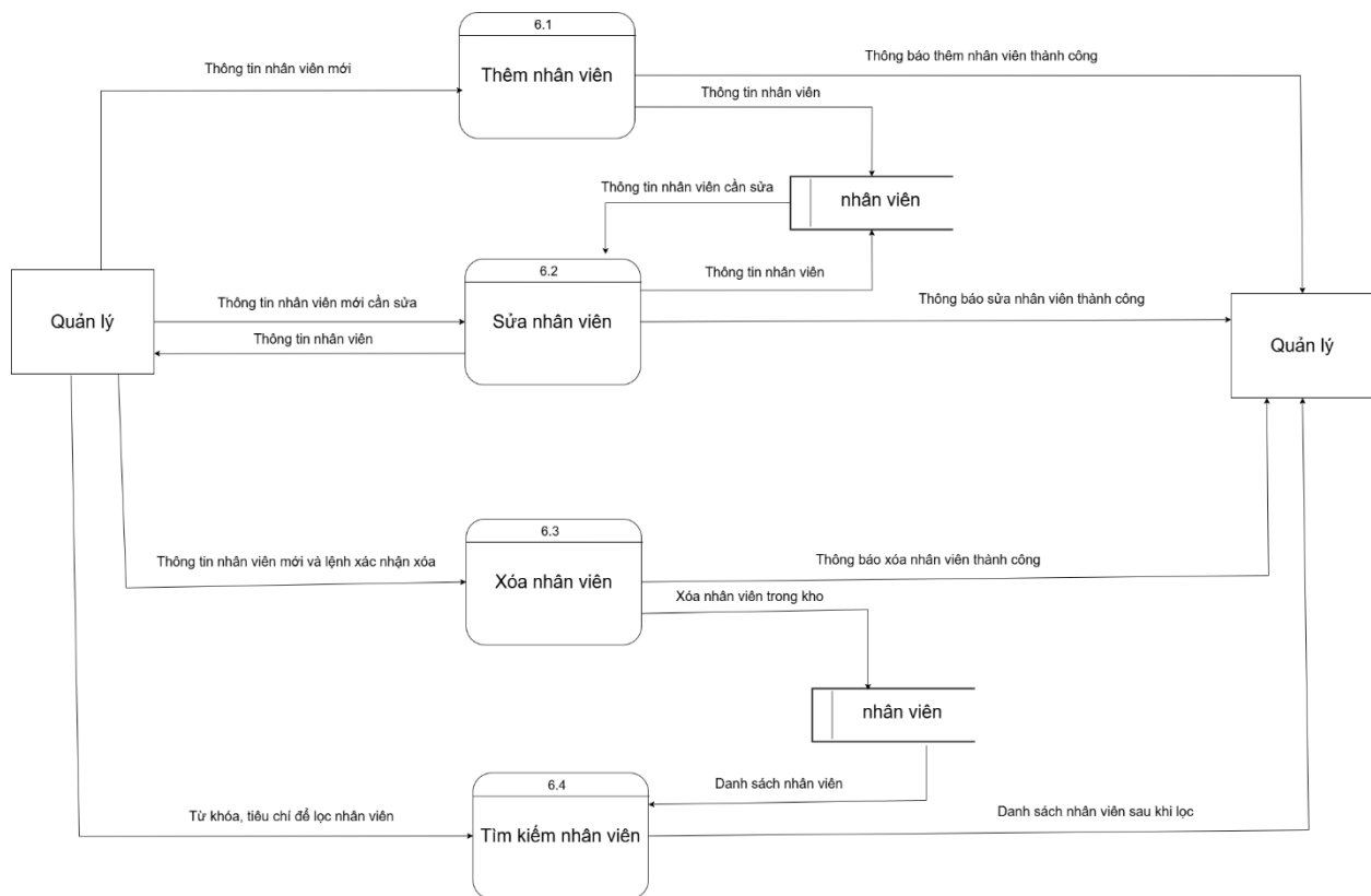
Hình 43. DFD quản lý nhân viên mức 2
