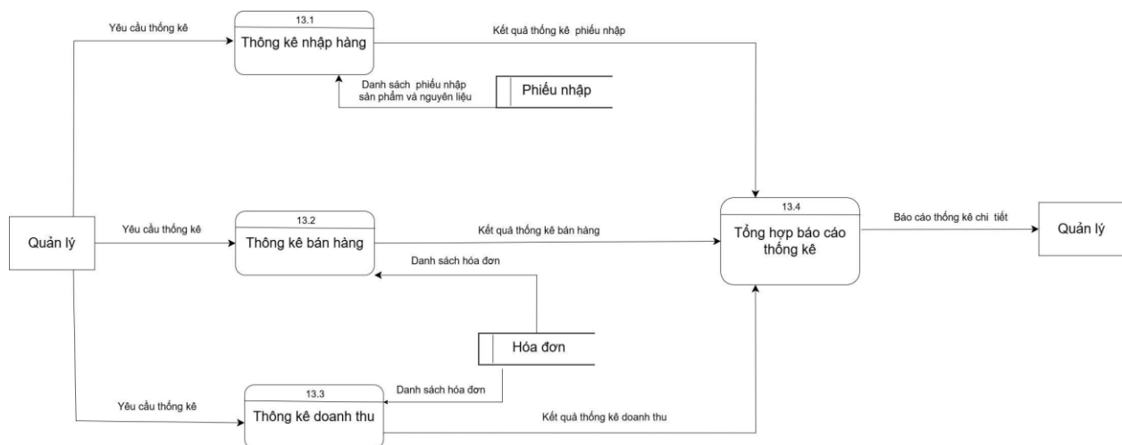
Hình 57. DFD thống kê ở mức 2
