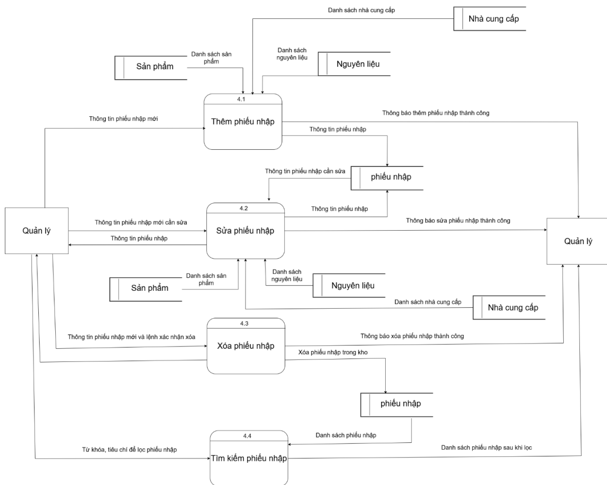
Hình 39. DFD Quản lý nhập kho mức 2
