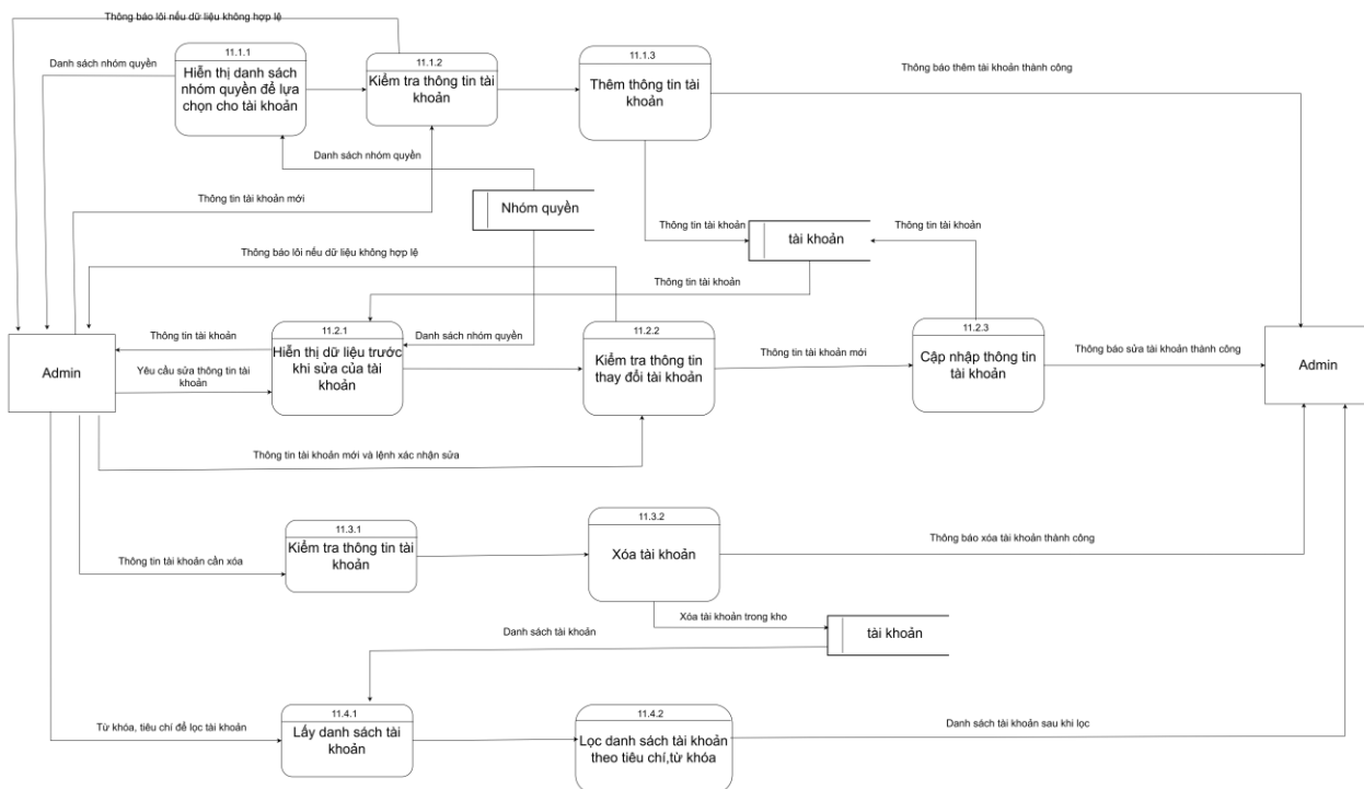
Hình 54. DFD Quản lý tài khoản ở mức 3
