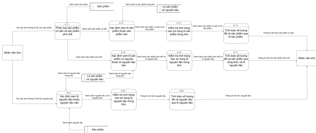
Hình 36. DFD Quản lý tồn kho mức 3
