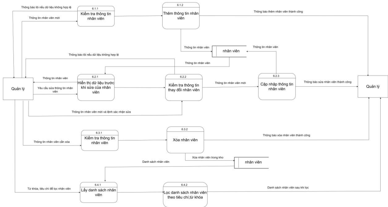
Hình 44. DFD quản lý nhân viên mức 3
