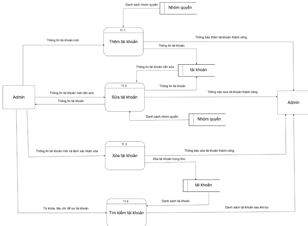
Hình 53. DFD Quản lý tài khoản ở mức 2
