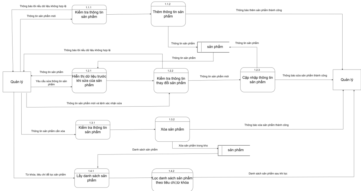
Hình 34. DFD quản lý sản phẩm mức 3
