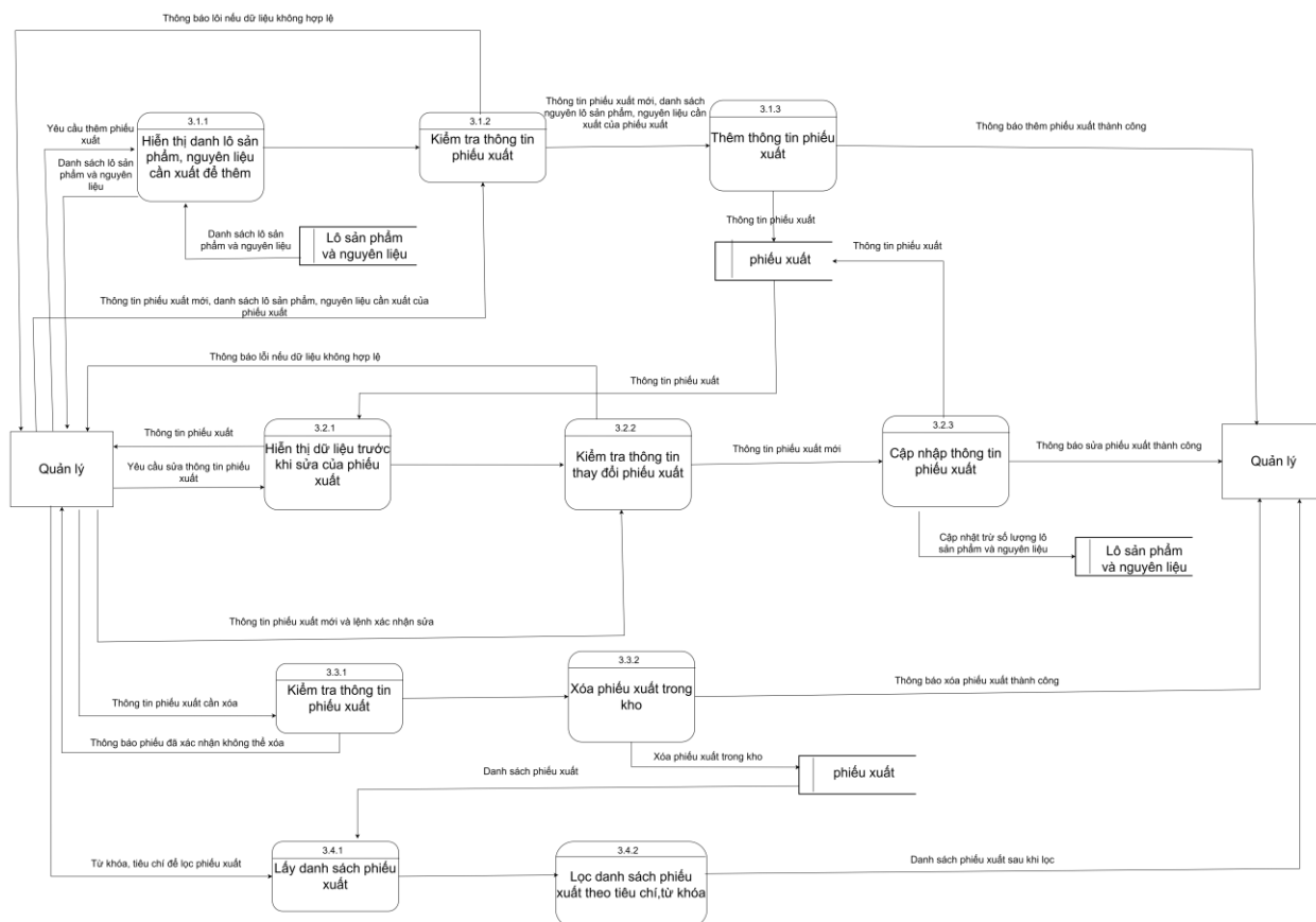
Hình 38. DFD Quản lý xuất kho mức 3
