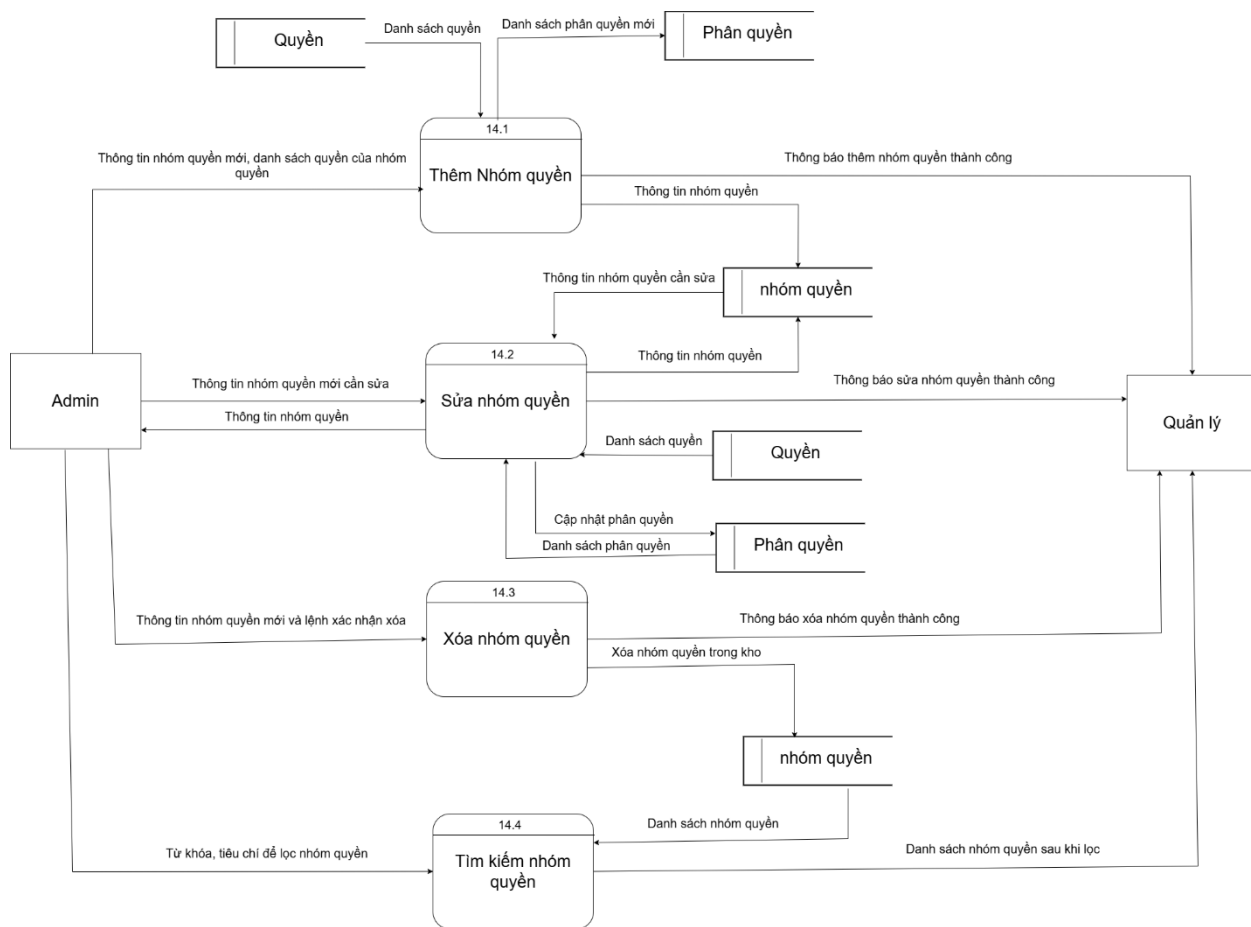
DFD Quản lý nhóm quyền ở mức 3:
