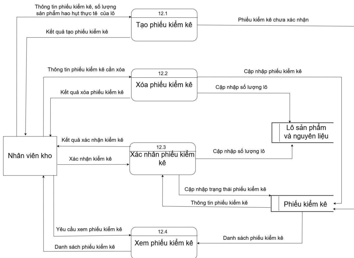
Hình 55. DFD quản lý kiểm kê ở mức 2
