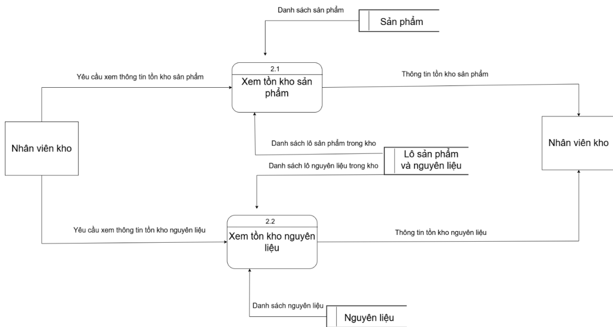
Hình 35. DFD quản lý tồn kho mức 2
