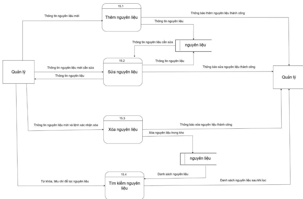
Hình 60. DFD quản lý nguyên liệu mức 2
