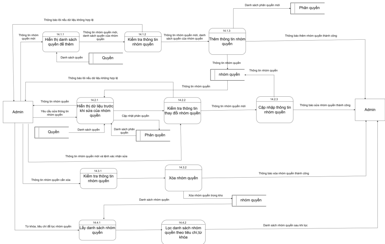
Hình 59. DFD Quản lý nhóm quyền ở mức 3
