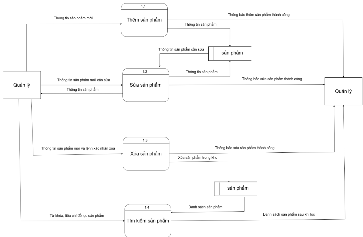
Hình 33. DFD quản lý sản phẩm mức 2
