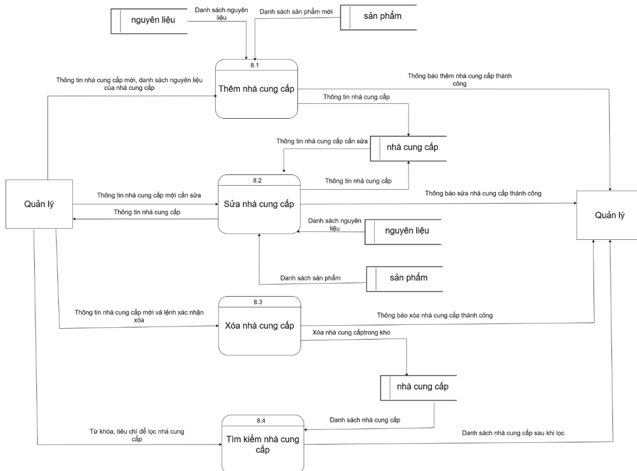
Hình 47. DFD quản lý nhà cung cấp mức 2
