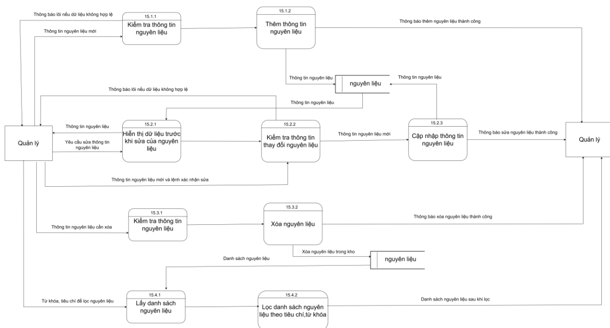
Hình 61. DFD Quản lý nguyên liệu mức 3
