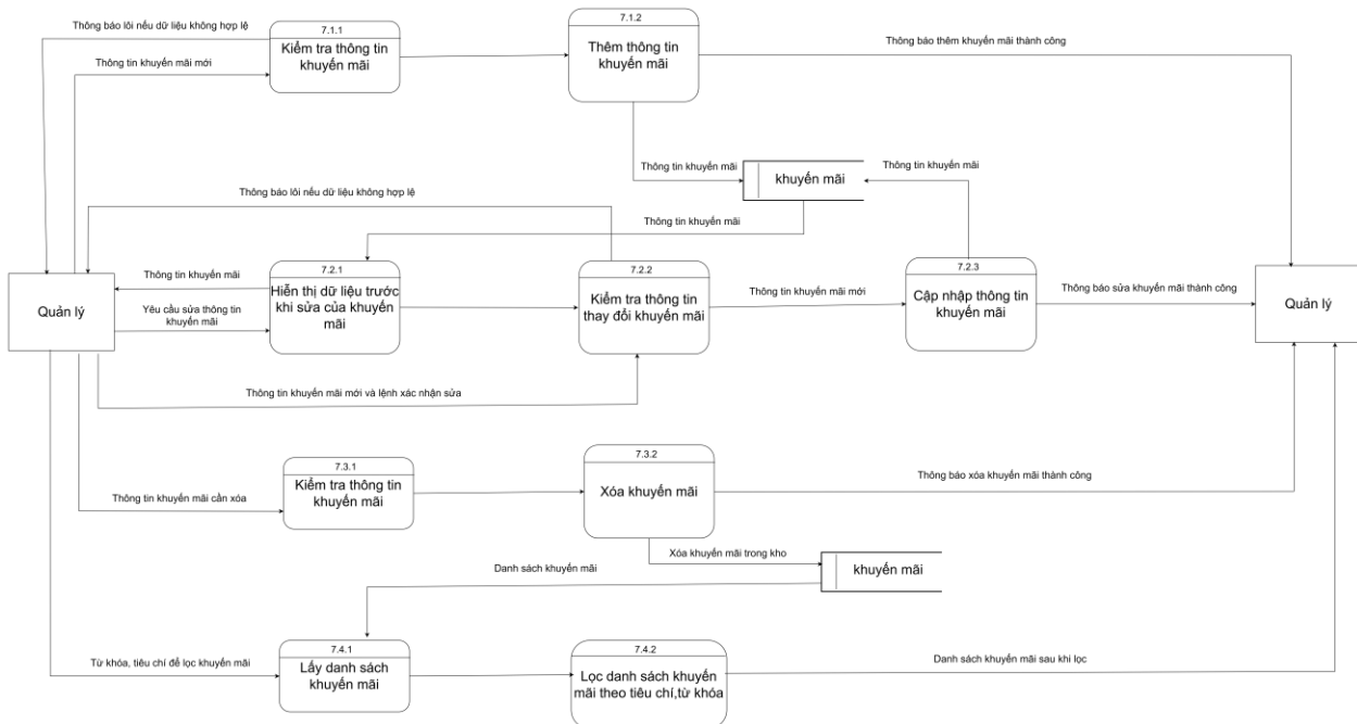
Hình 46. DFD quản lý khuyến mãi mức 3
