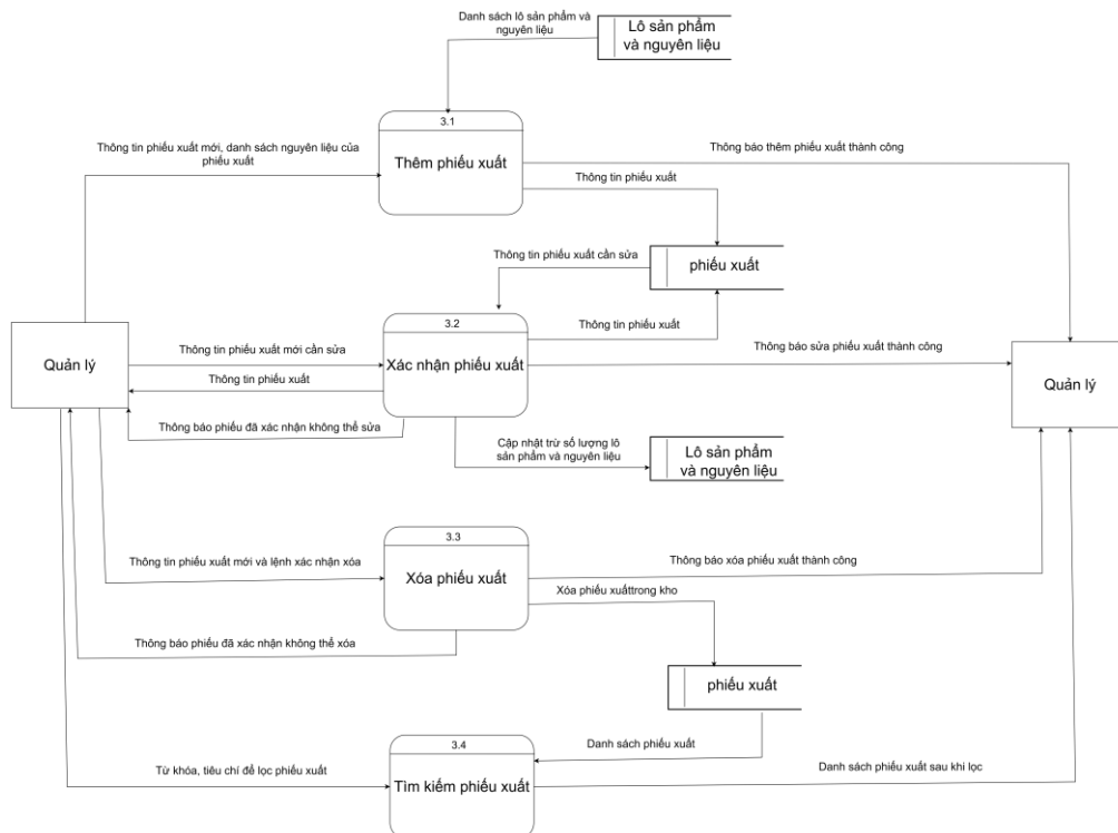
Hình 37. Quản lý xuất kho mức 2
