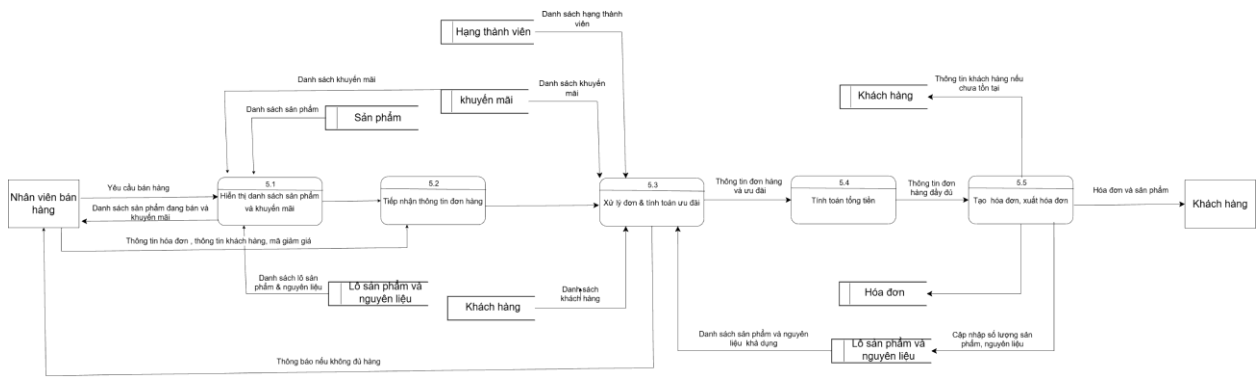
Hình 41. DFD Quản lý bán hàng mức 2
