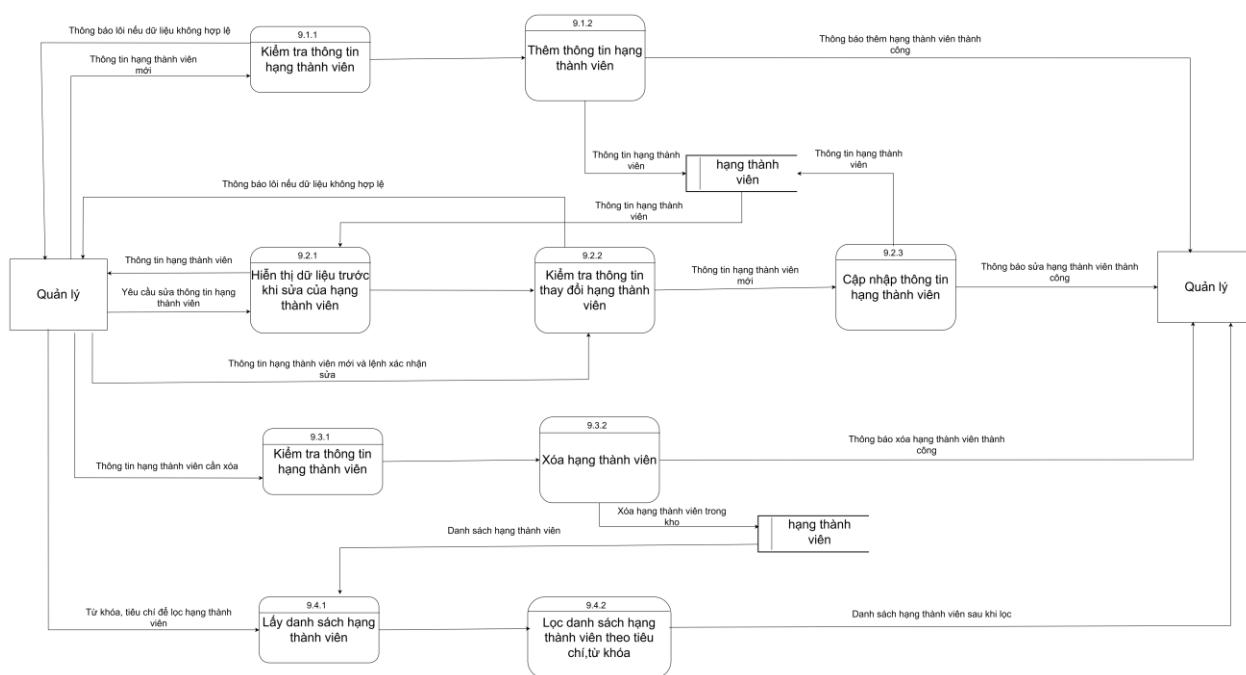
Hình 50. DFD quản lý hạng thành viên mức 3
