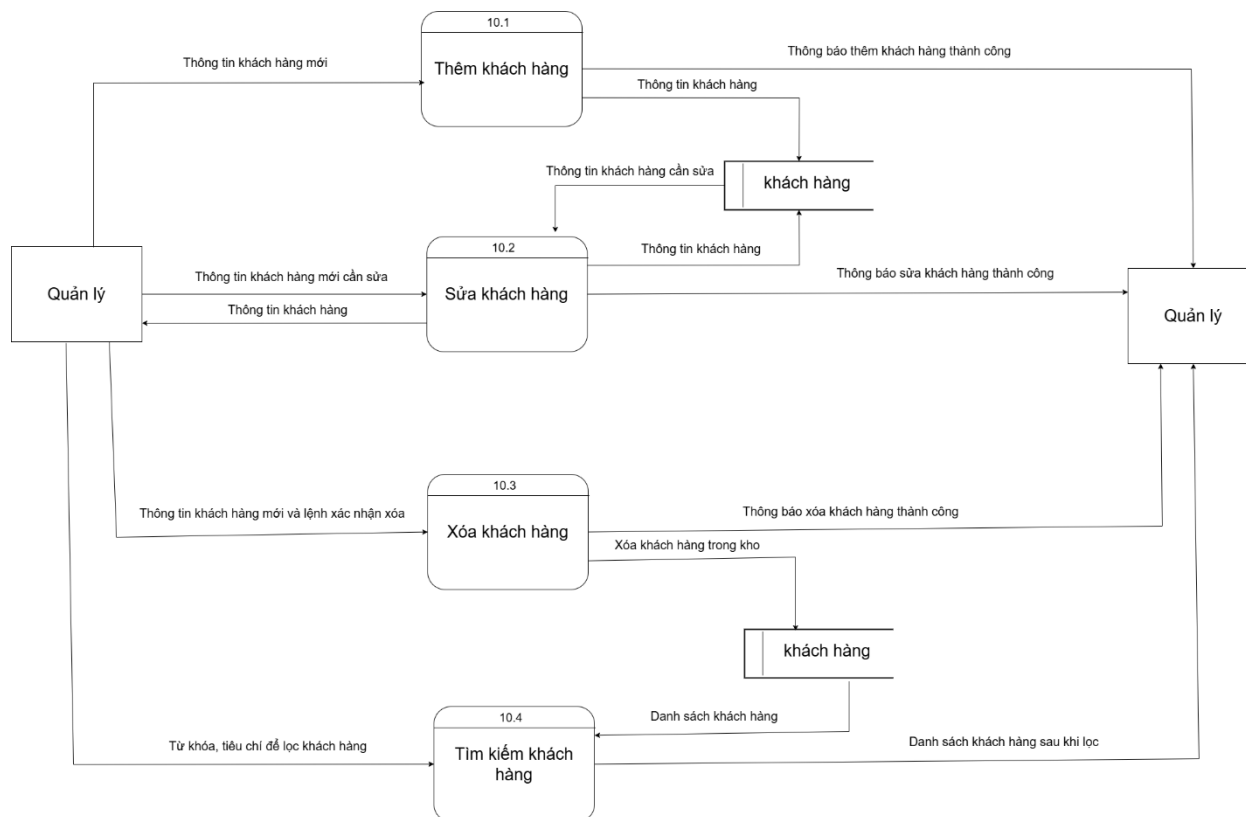
Hình 51. DFD quản lý khách hàng mức 2
