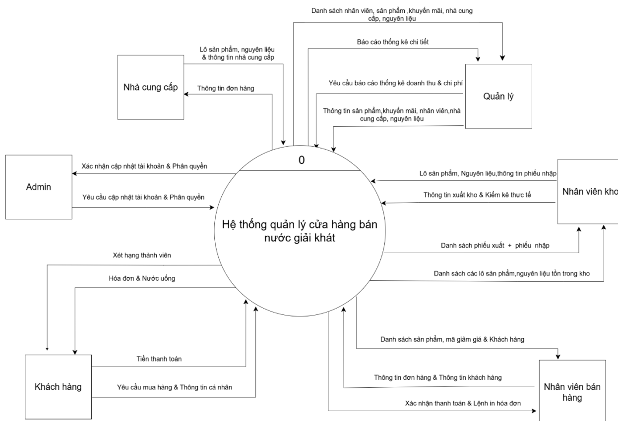
Hình 31. DFD mức quan niệm
