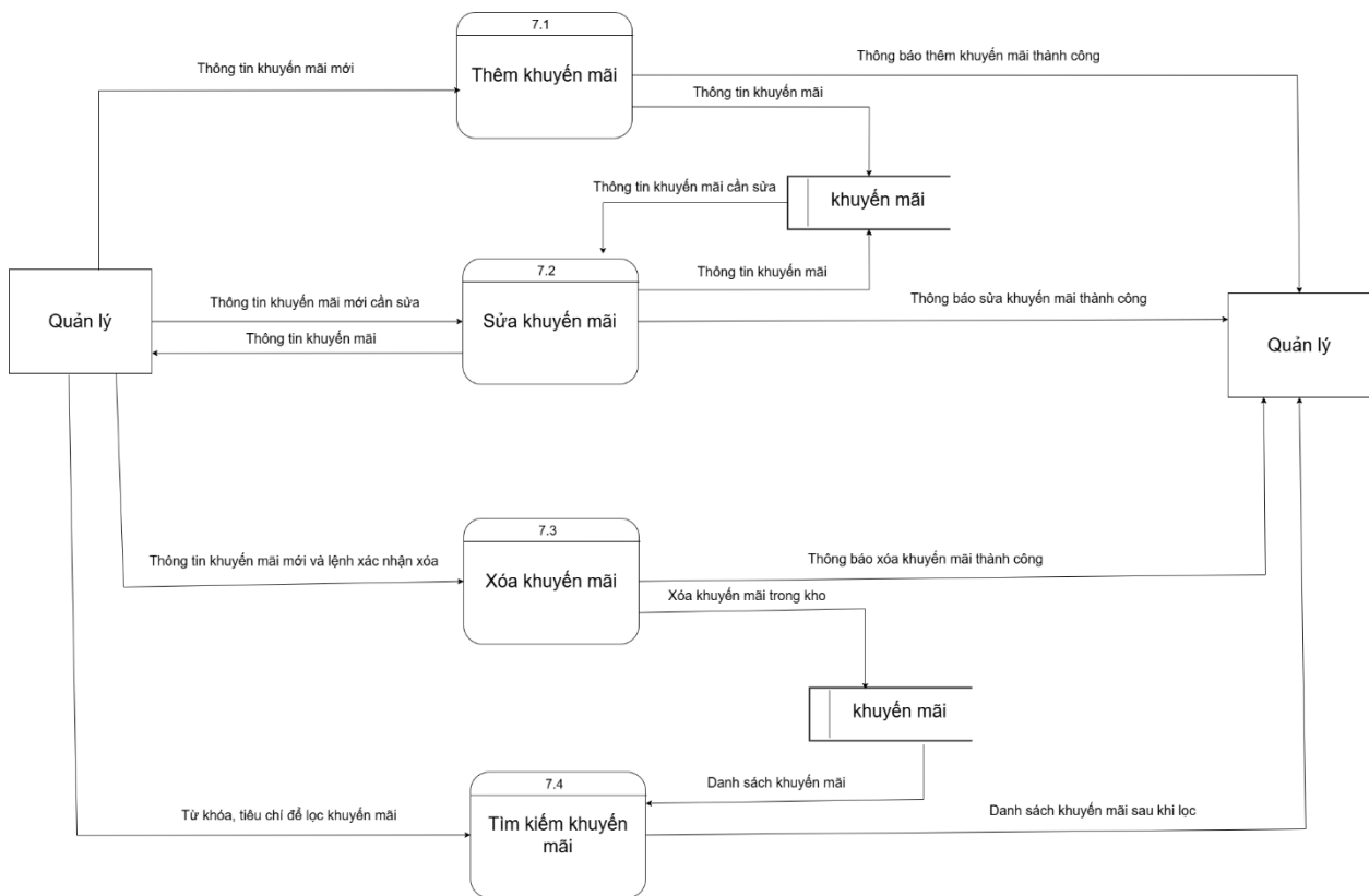
Hình 45. DFD quản lý khuyến mãi mức 2
