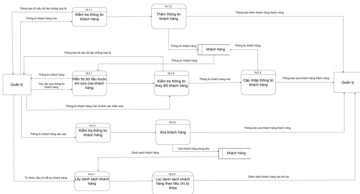
Hình 52. DFD quản lý khách hàng mức 3
