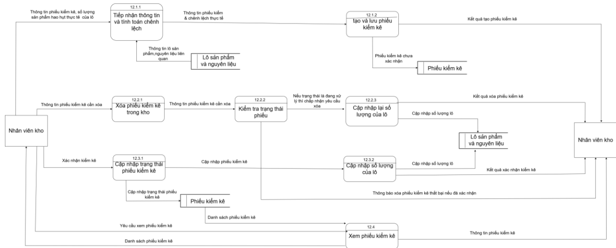
Hình 56. DFD Kiểm kê ở mức 3
