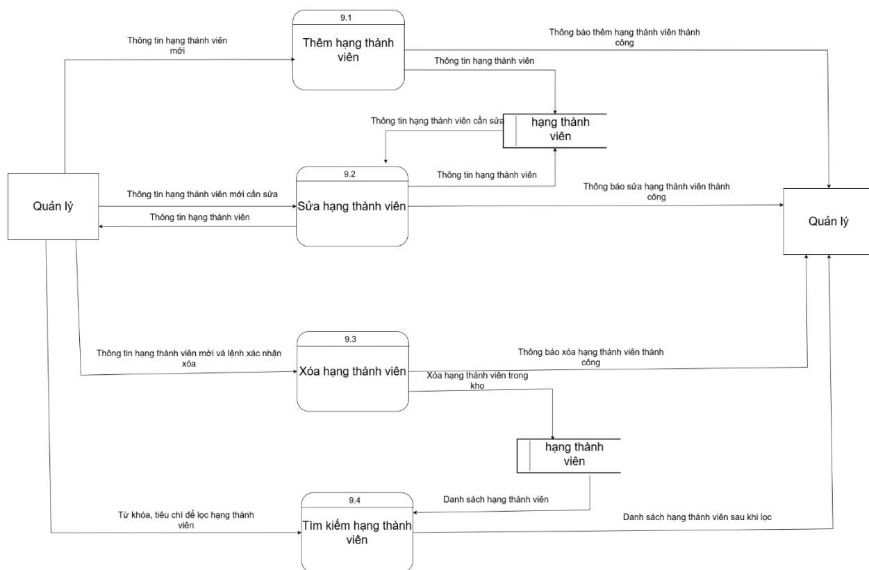
Hình 49. DFD quản lý hạng thành viên mức 2
