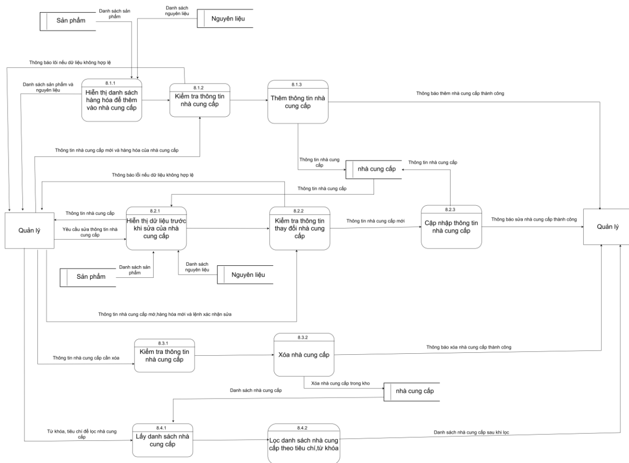
Hình 48. DFD quản lý nhà cung cấp mức 3
