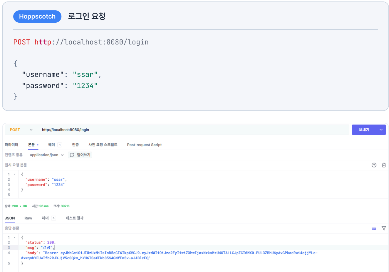
그림 4-14. 로그인 응답
