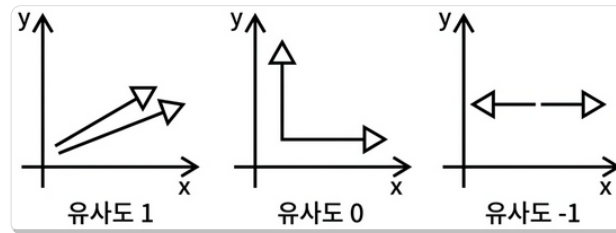
그림 0-8: 코사인 유사도의 각도에 따른 값의 변화
