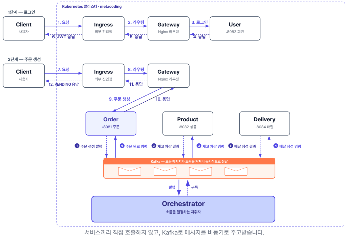
그림 4-1. 챕터 4 한눈에 보기 - 서비스-Orchestrator-Kafka 3층 구조
