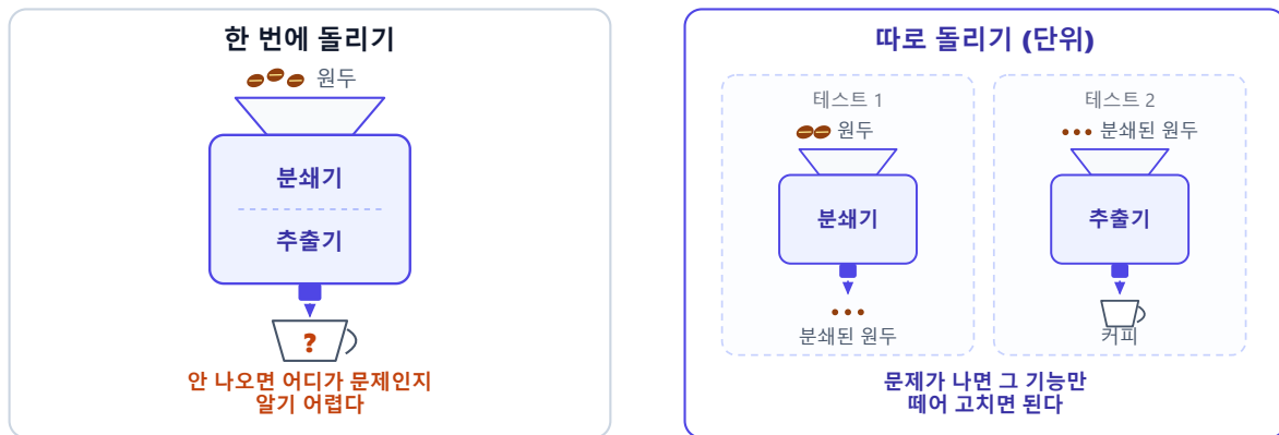
그림 2-26. 단위 테스트가 필요한 이유
