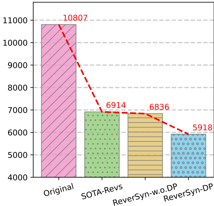
GPT
