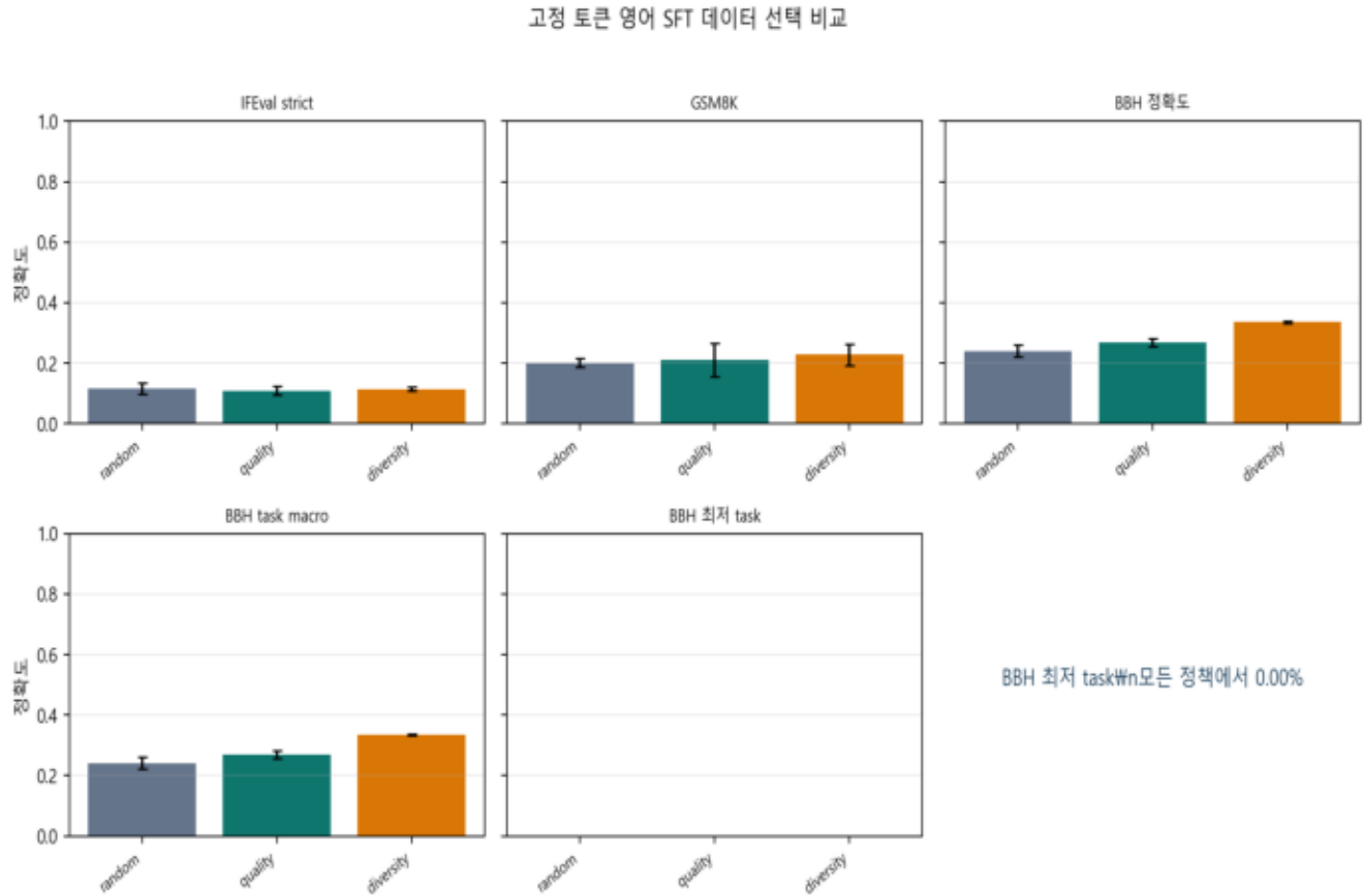
그림 1. 전략별 평가 비교. 고정 evaluation subset의 평균과 seed 표준편차입니다. 정확한 값은 원고의 표와 CSV 결과를 확인하십시오.
