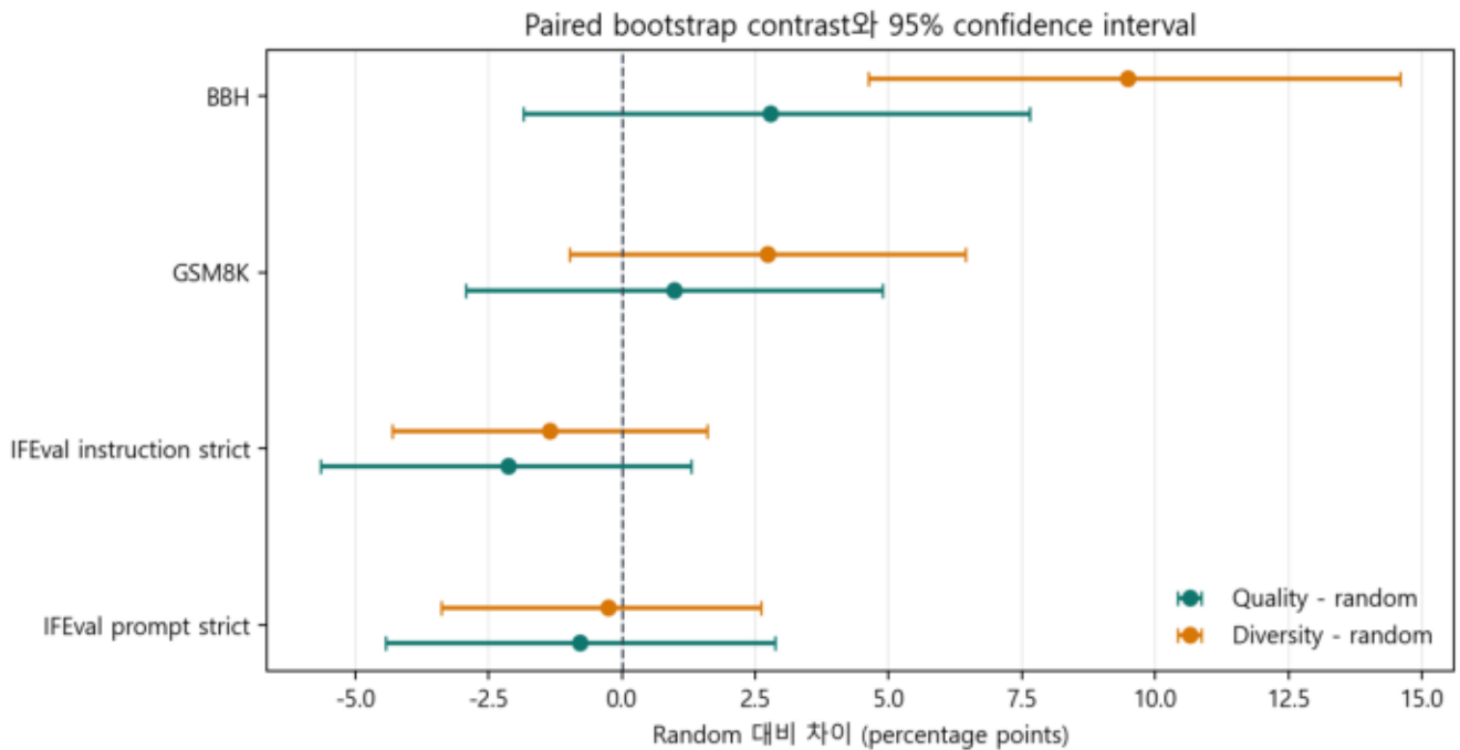
그림 2. Random 기준 paired bootstrap contrast입니다. 점은 효과 추정치이고 선은 95% confidence interval입니다.
