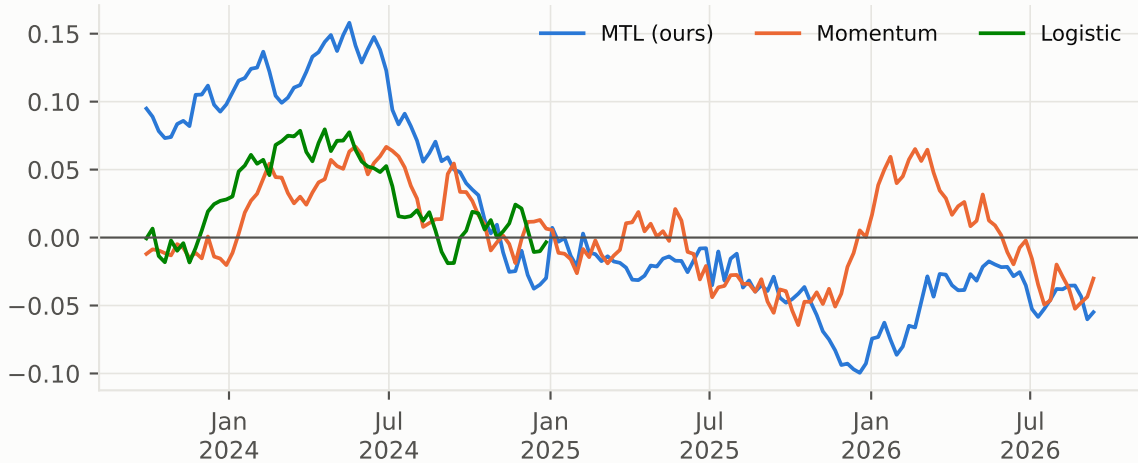
Rolling 26w rank-IC
