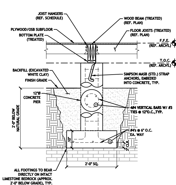
PIER & BEAM, TYP. TYPE F1 ③
