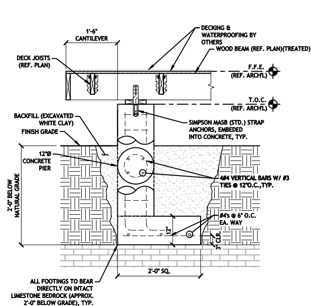
PIER & BEAM, TYP. ④
