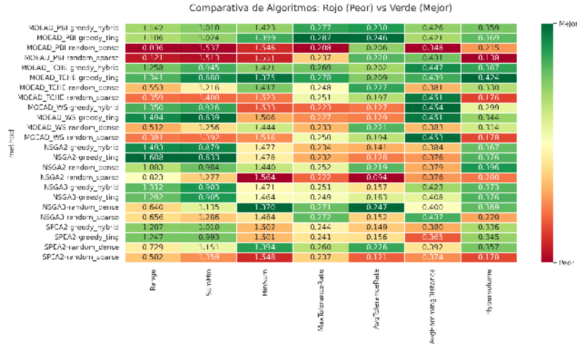
Figura 7: Comparativa de métricas para la Ejecución A.
