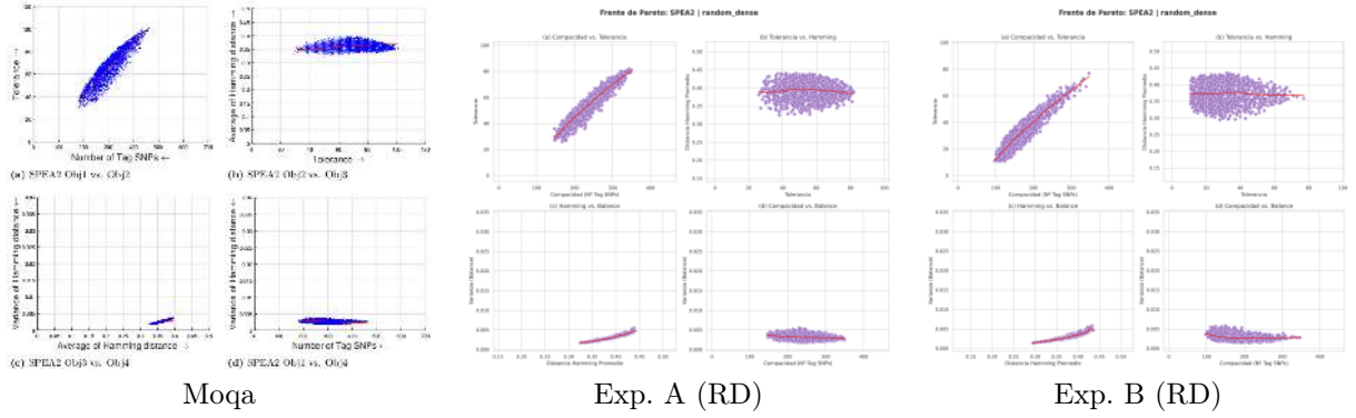
Figura 17: Comparativa de frentes Random para SPEA2 frente al original de Moqa.
