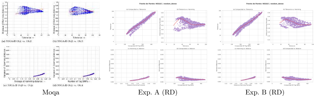
Figura 15: Comparativa de frentes Random para NSGA-II frente al original de Moqa.
