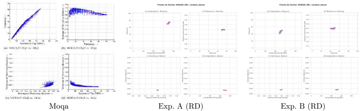
Figura 21: Comparativa de frentes Random para MOEA/D-PBI frente al original de Moqa.
