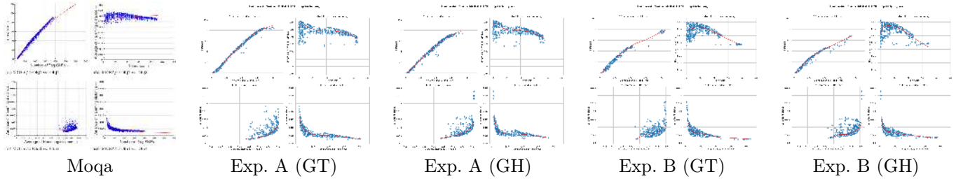
Figura 22: Comparativa de frentes Greedy para MOEA/D-TCHE frente al original de Moqa.
