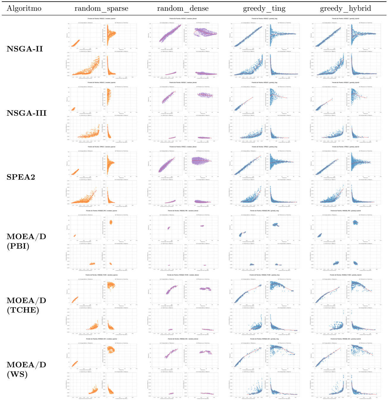
Cuadro 16: Galería de Frentes de Pareto (B)
