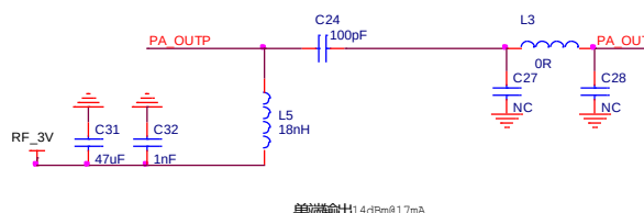
图 7: 单端输出的配置
