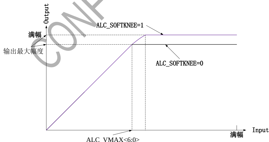
图 5：ALC 示意图（拐点幅度大）
