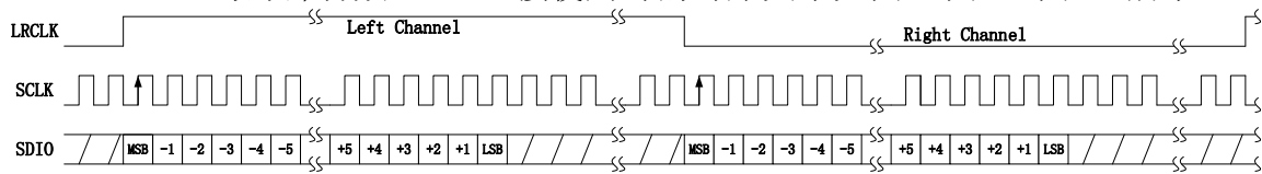
图 11: KT1607 与外部音频 DAC 连接工作在左对齐方式时序图
