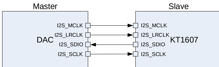
图 10: KT1607 作为从及输出与外部音频 DAC 连接示意图
