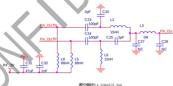
图 6: 差分输出的配置
