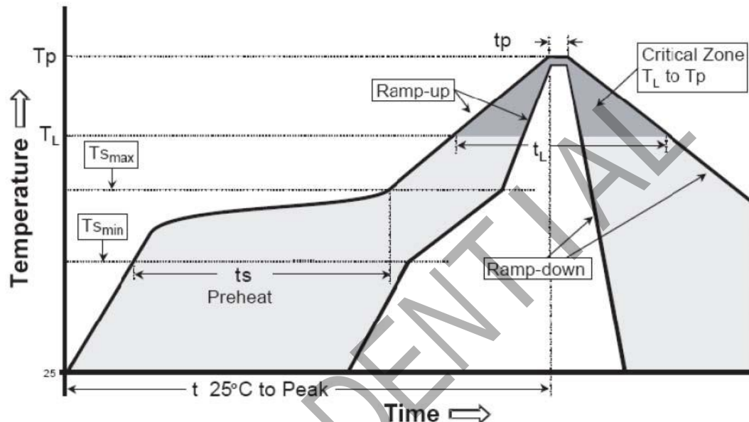
图 20: 典型回流焊曲线
