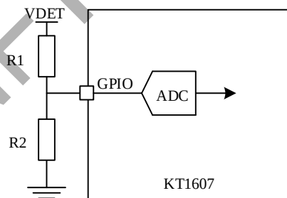
图 15：电压检测连接示意图
