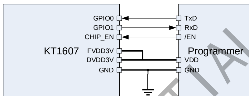
图 14: KT1607 与烧录器连接示意图
