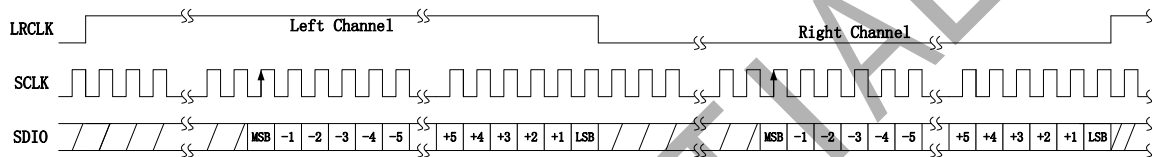
图 13: KT1607 与外部音频 DAC 连接工作在右对齐方式时序图
