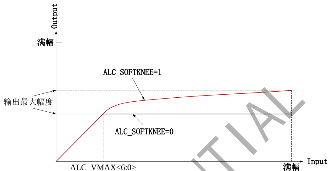
图 4：ALC 示意图（拐点幅度小）
