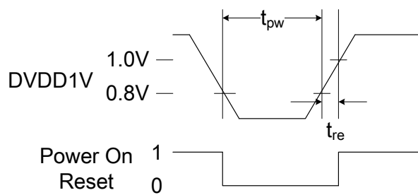
图 1：上电复位时序图
