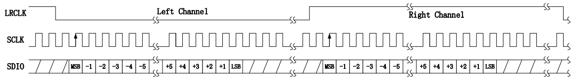
图 12: KT1607 与外部音频 DAC 连接工作在 I 2 S 方式时序图
