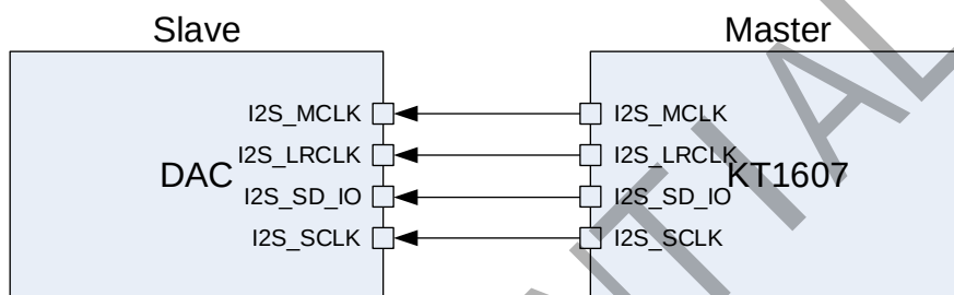
图 9: KT1607 作为主及输出与外部音频 DAC 连接示意图
