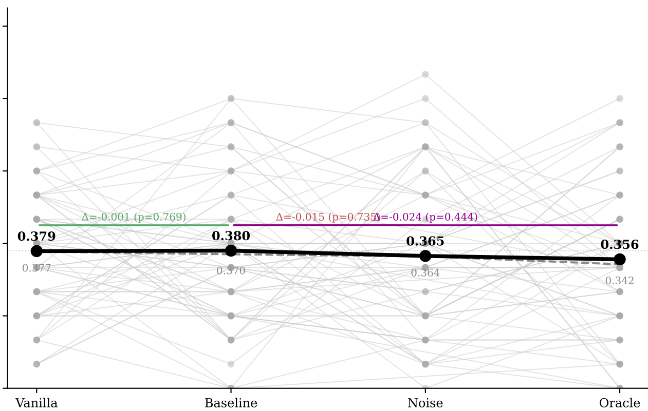
OLMo
