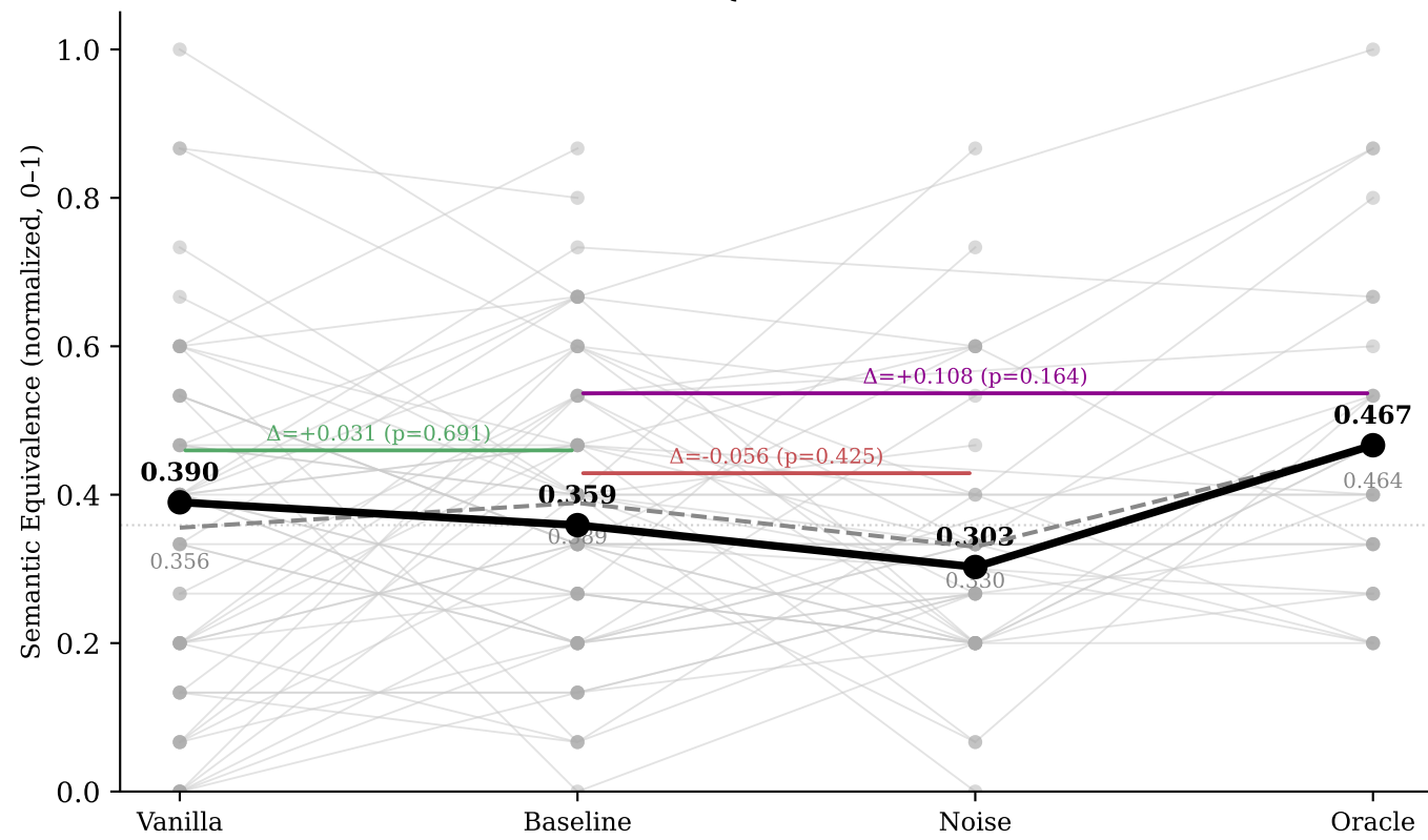
Qwen3
