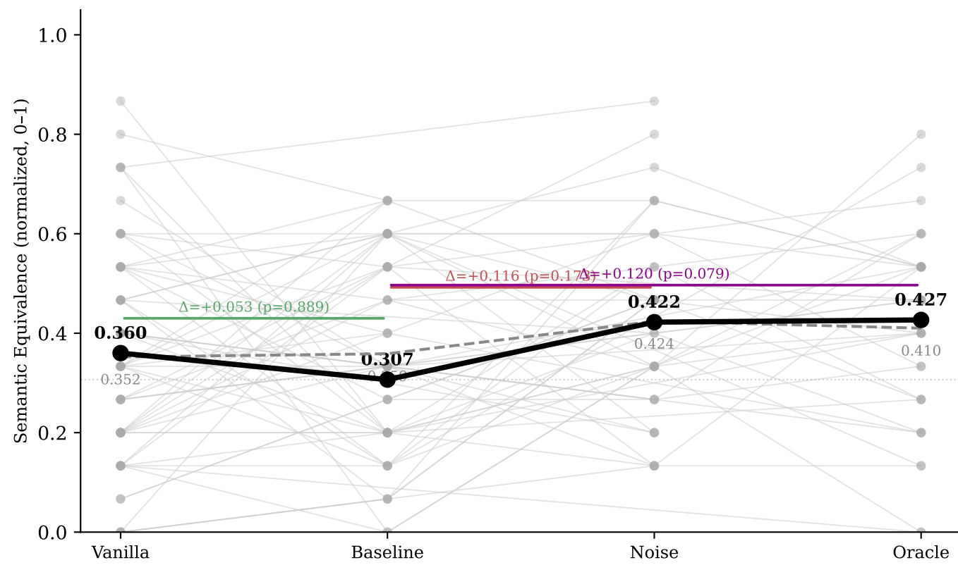
Qwen3
