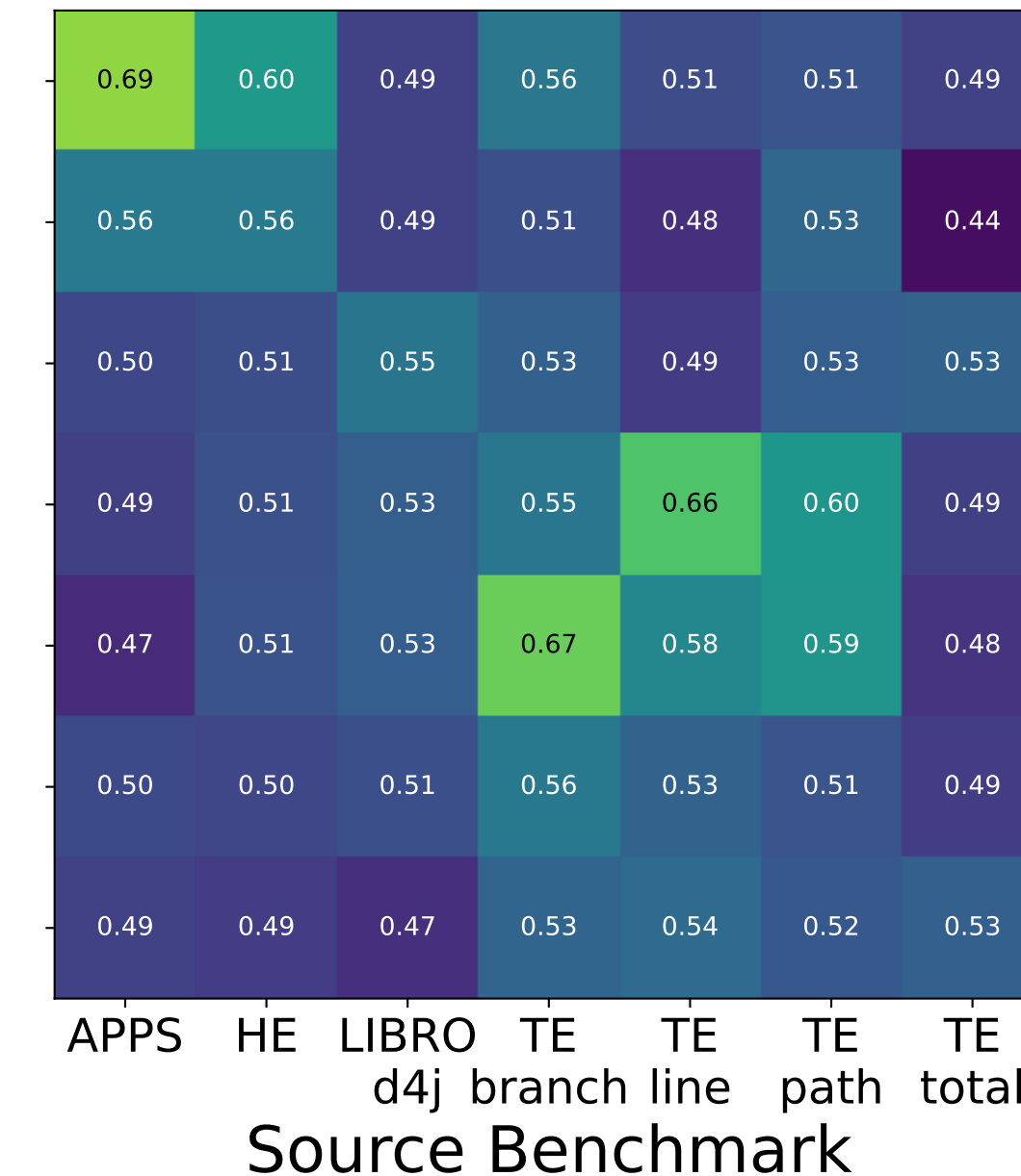
RouteLLM
