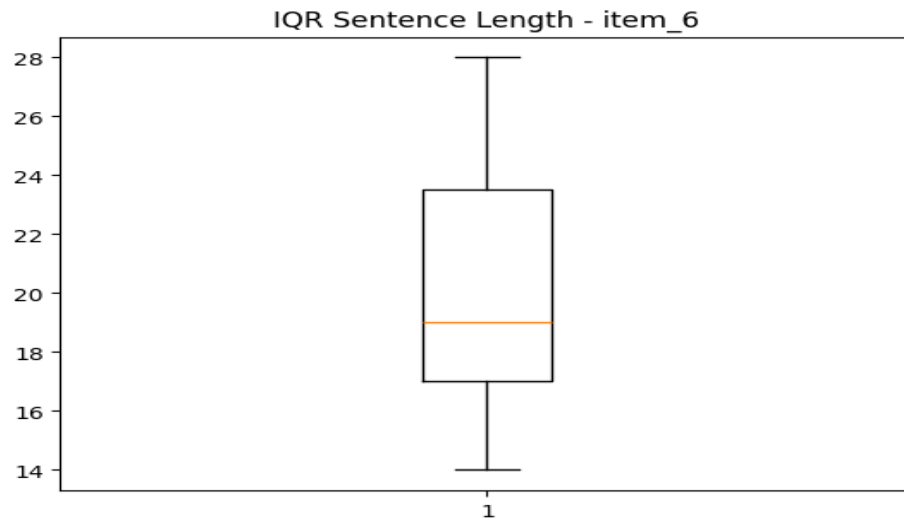
sentence_IQR_item_6.png
