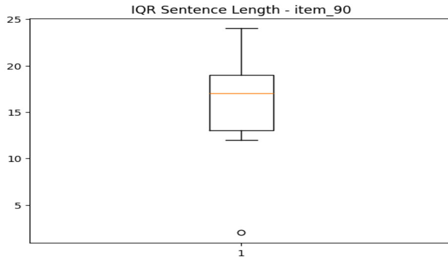
sentence_IQR_item_90.png
