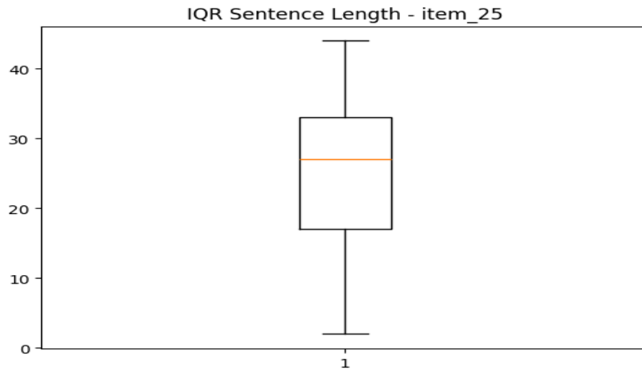
sentence_IQR_item_25.png
