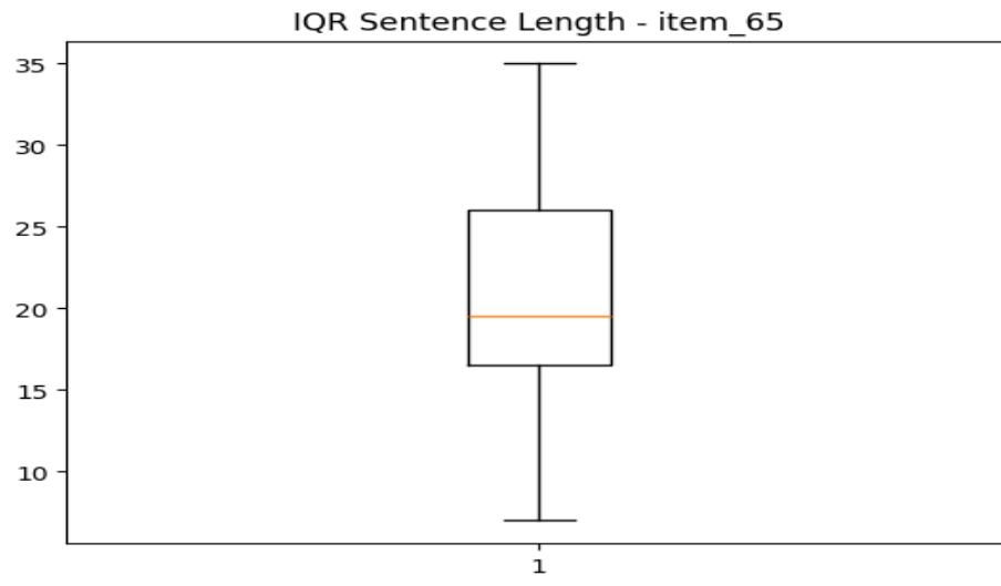
sentence_IQR_item_65.png
