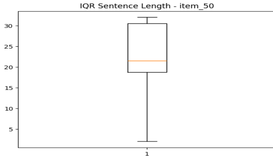
sentence_IQR_item_50.png
