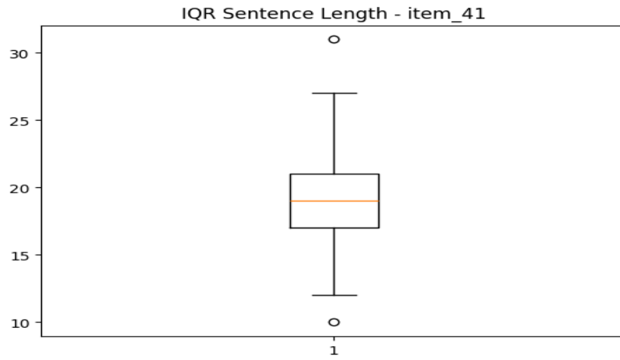
sentence_IQR_item_41.png
