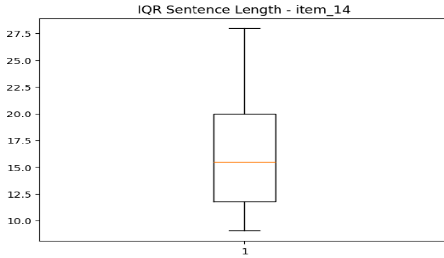
sentence_IQR_item_14.png
