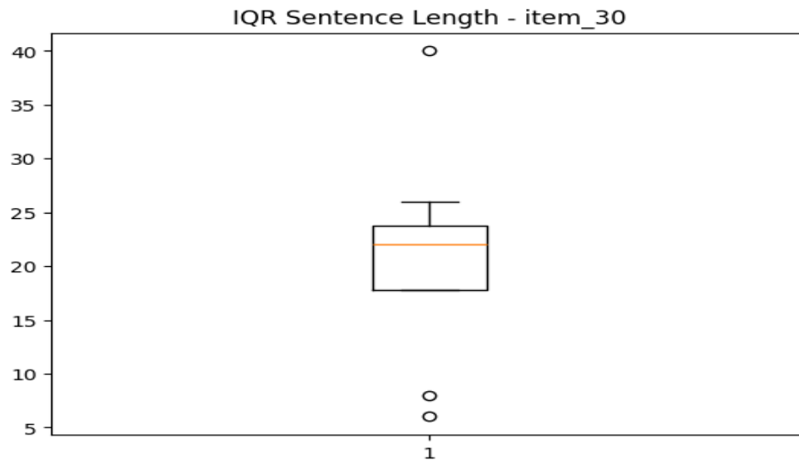
sentence_IQR_item_30.png
