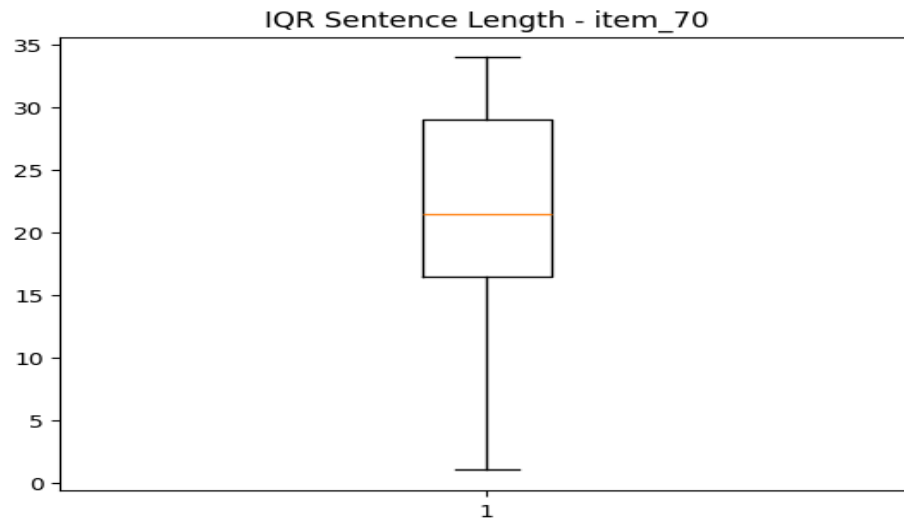
sentence_IQR_item_70.png
