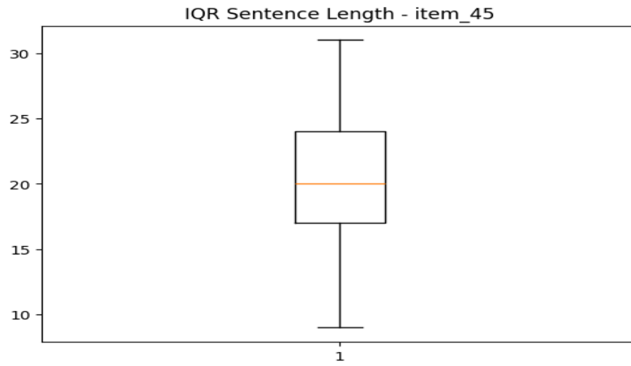
sentence_IQR_item_45.png
