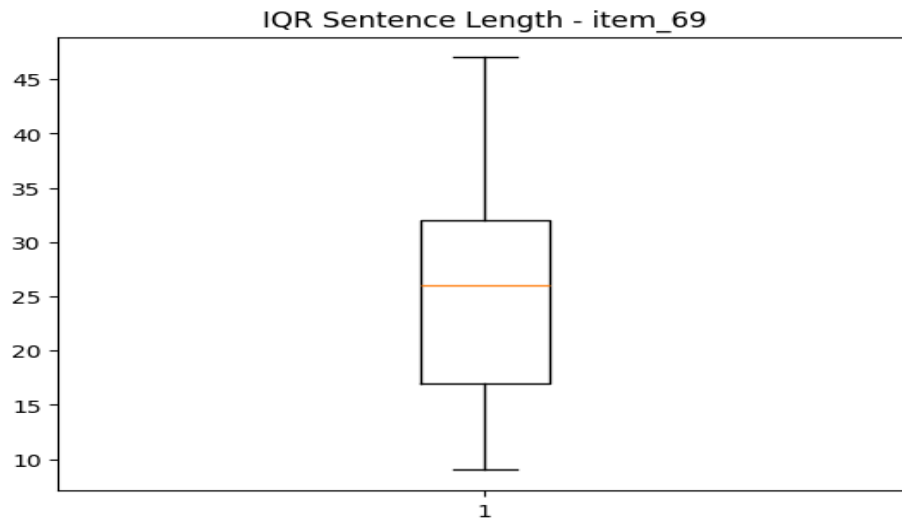
sentence_IQR_item_69.png
