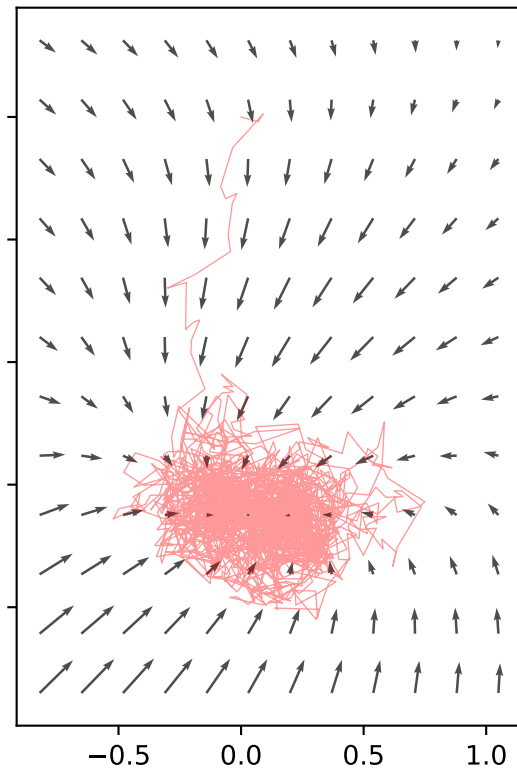
MC
