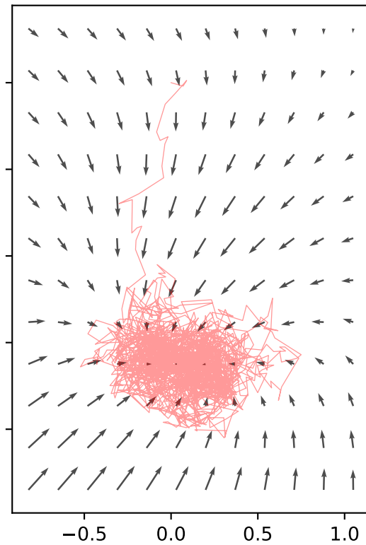
GMIX
