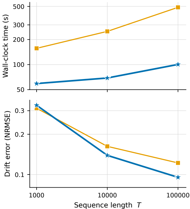
★ EFGP-SING ■ SparseGP (M=49)
