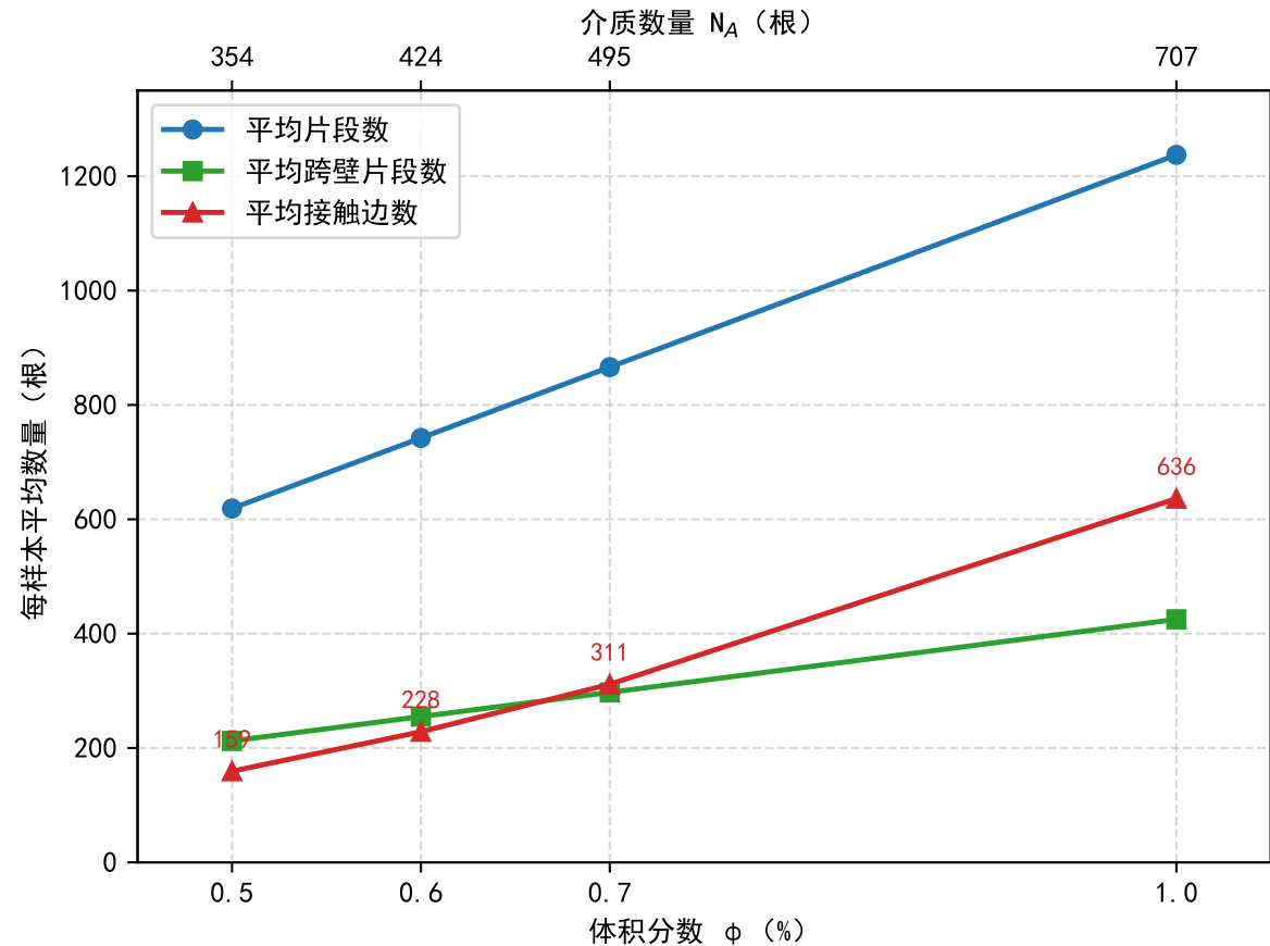
问题2：随机微构体几何统计量随体积分数变化（M=2000）
