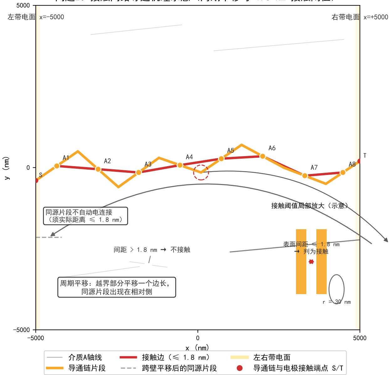
问题2：接触网络导通机理示意（周期平移与 1.8 nm 接触阈值）
