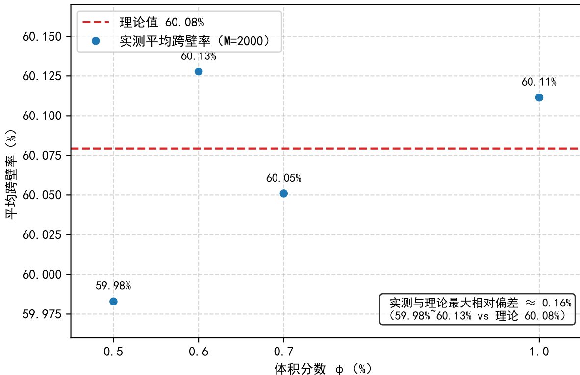
问题2：轴线跨壁率与理论值一致性验证 (M=2000)
