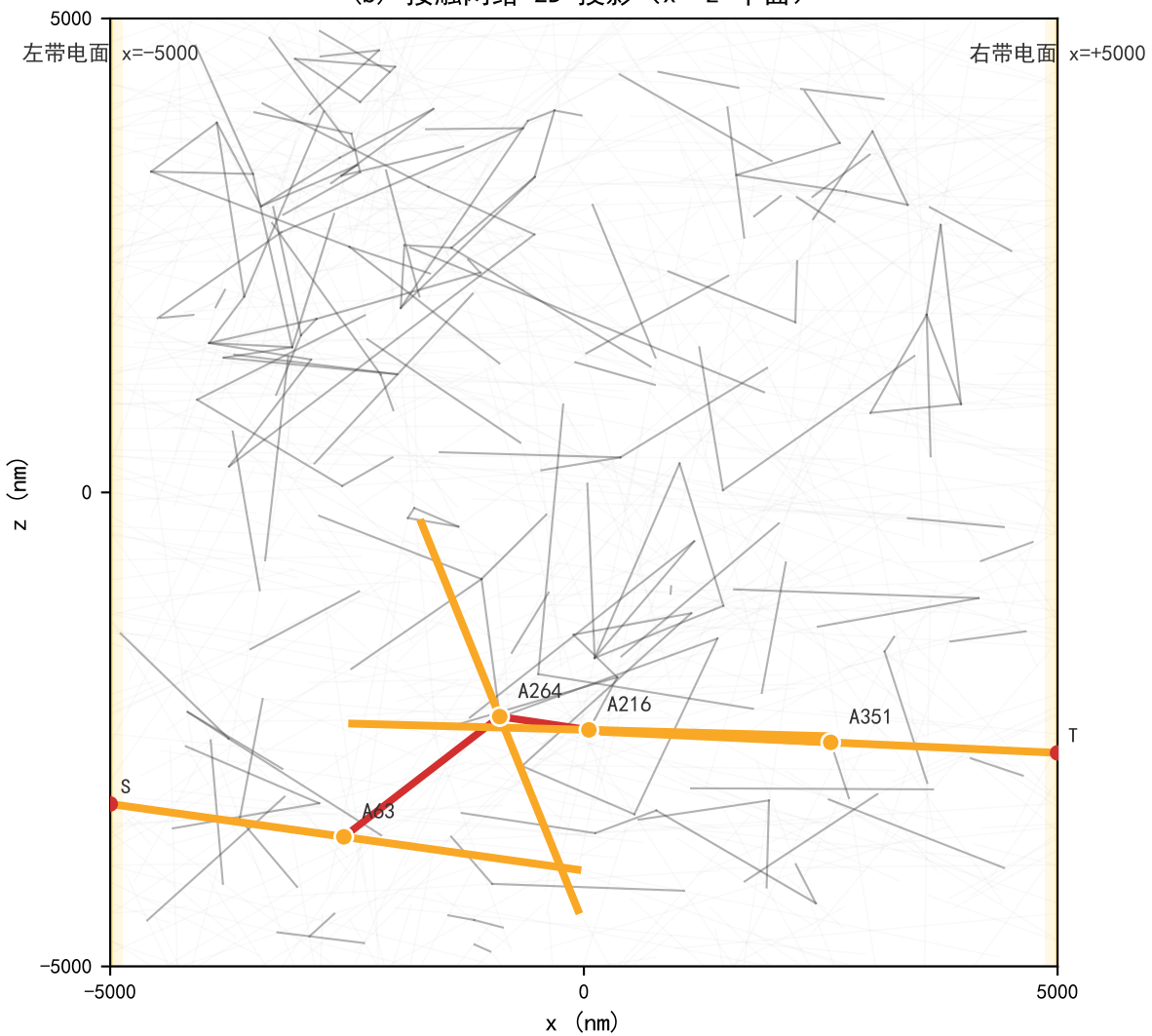
(b) 接触网络 2D 投影 ( x-z 平面)
