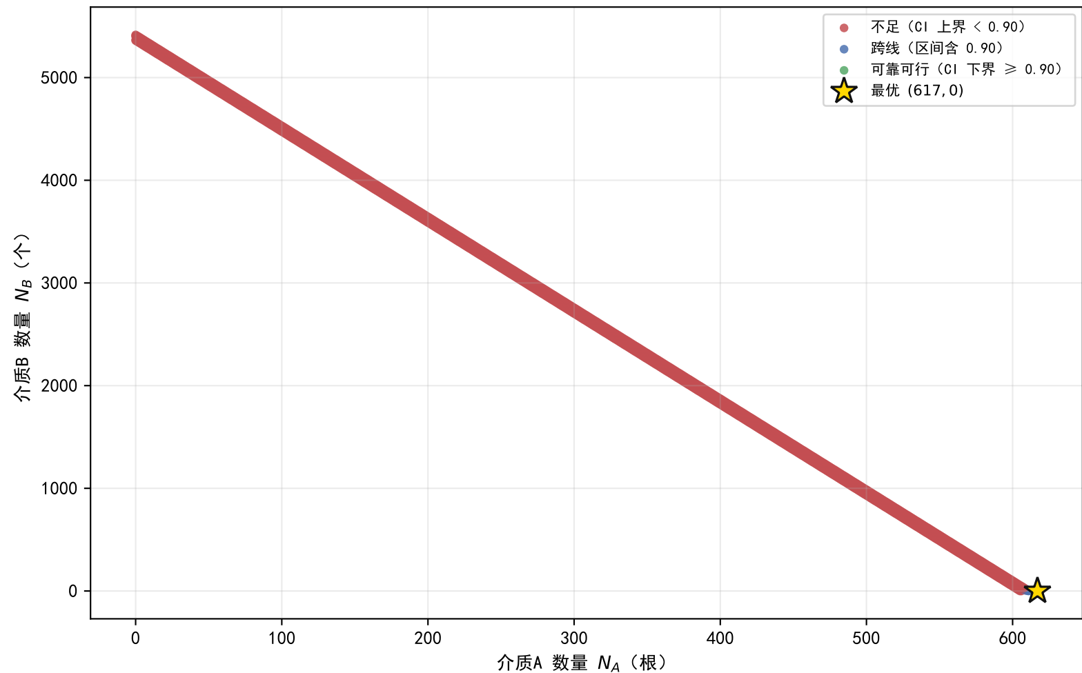
问题4：验证带边界点与非支配判定
