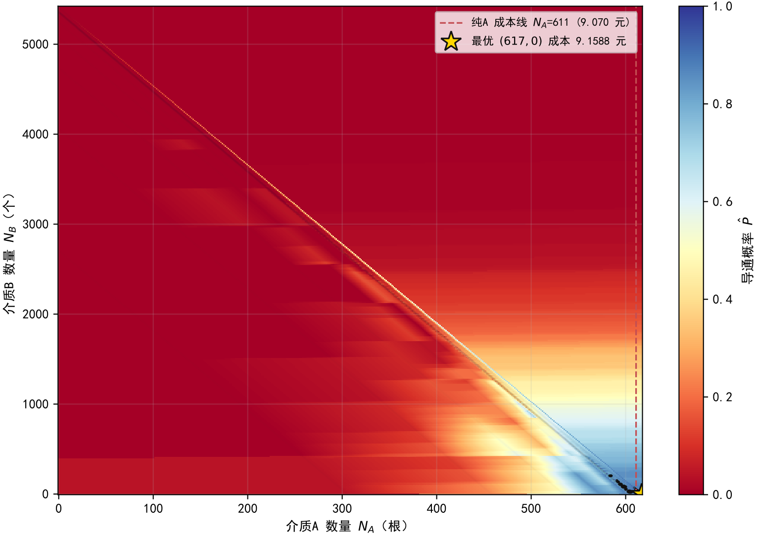
问题4：导通概率 \hat{P}(N_A, N_B) 热图与 90% 可行边界
