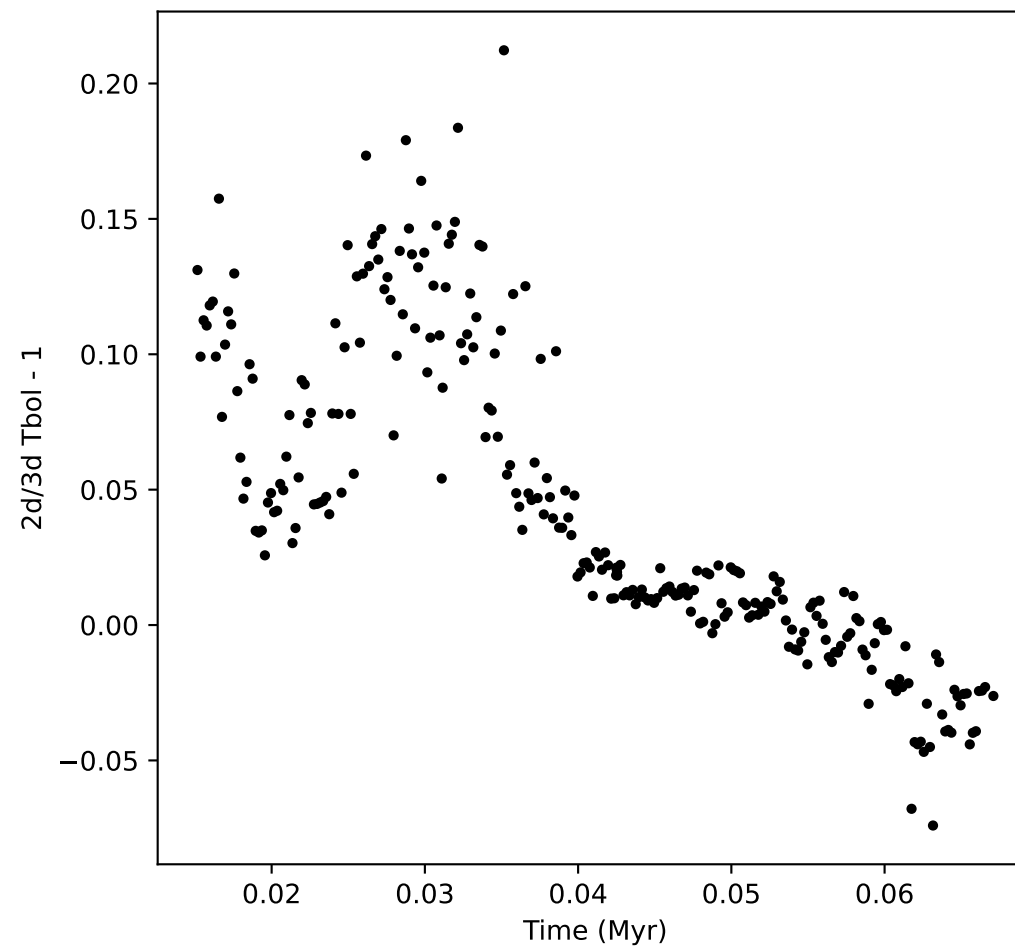
inclination 45
