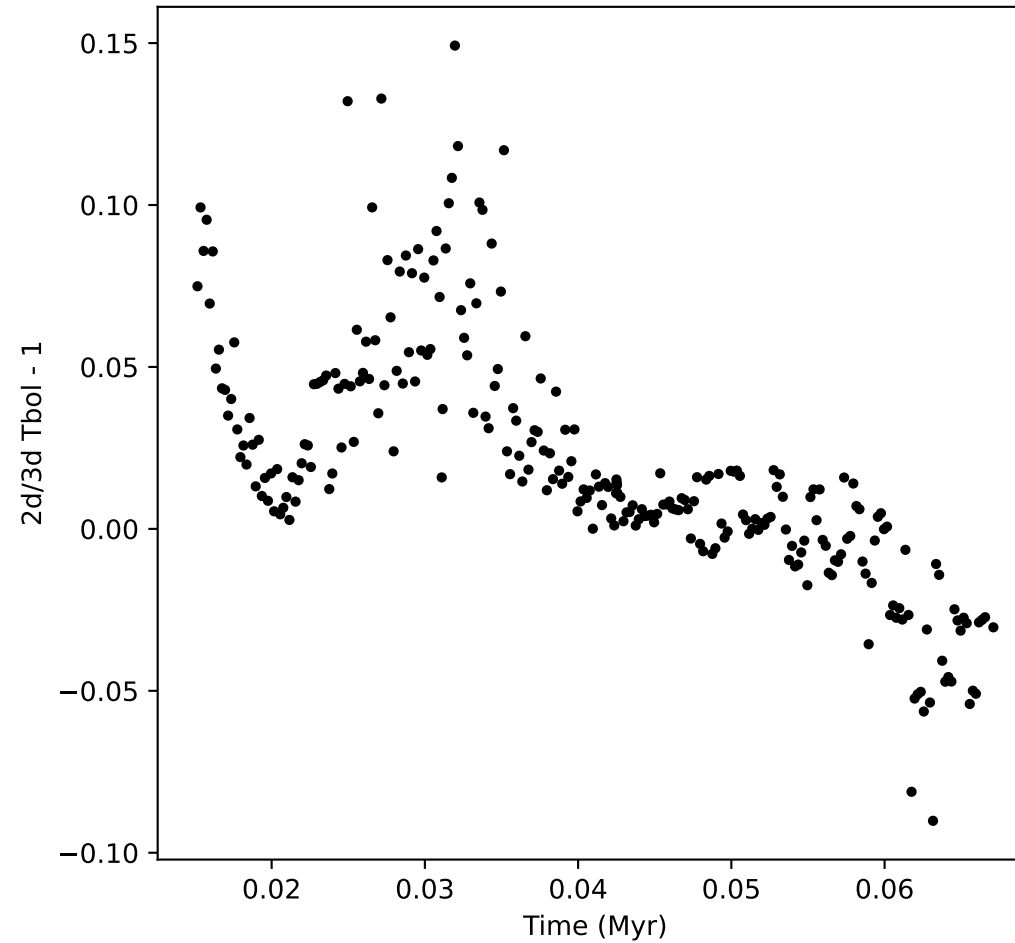
inclination 75
