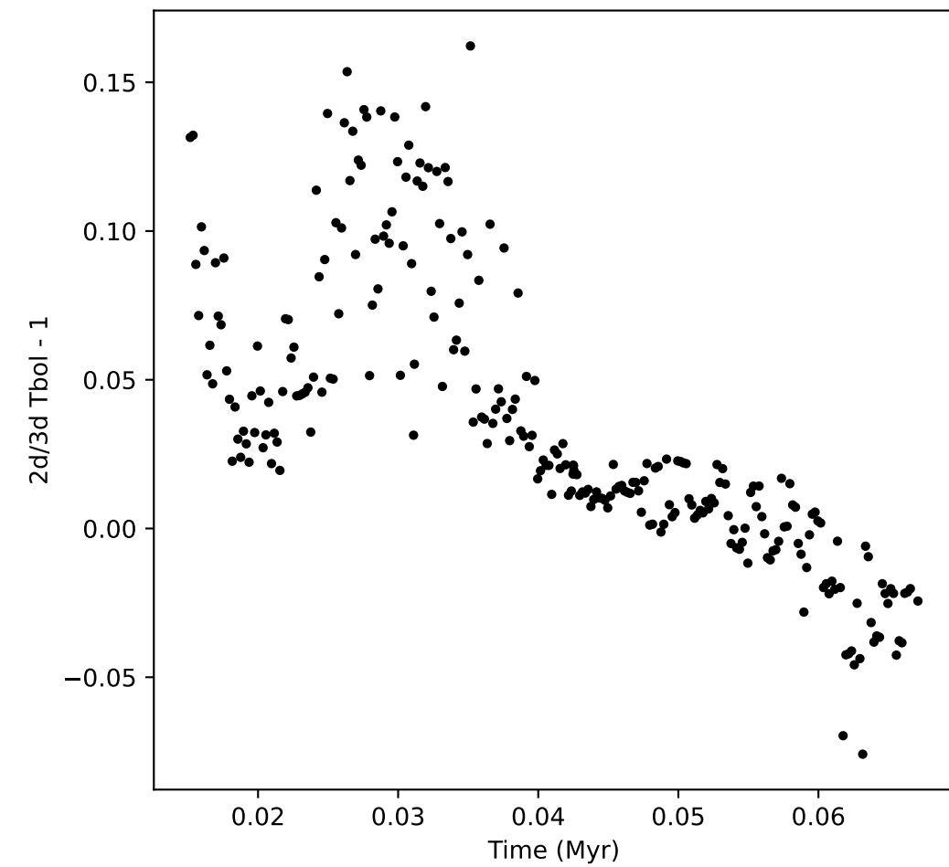
inclination 55
