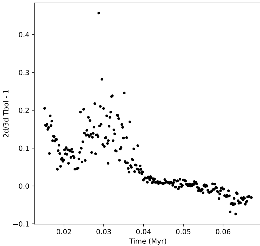
inclination 35
