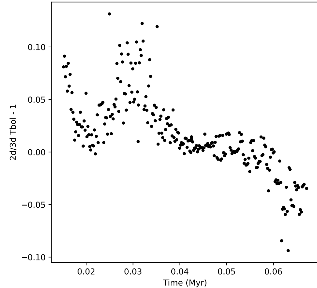
inclination 85
