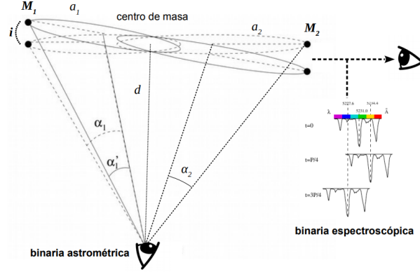
Figura 7: Binaria espectroscópica.
