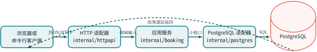
图 12.1 SeatKeeper 第一版请求路径
