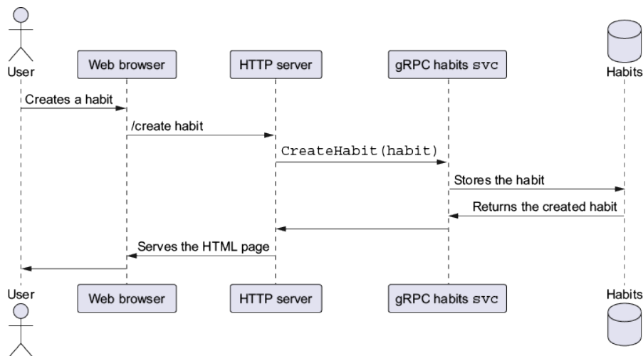
图 11.1 系统总体架构的 UML 图
