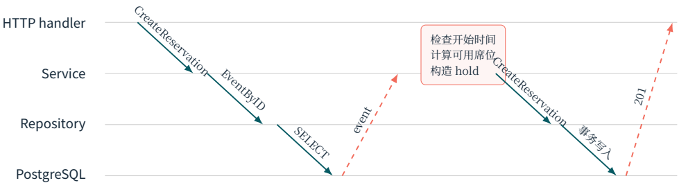
图 12.2 创建占座的调用顺序
