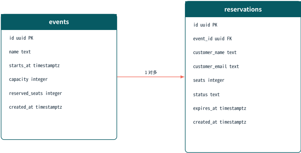
图 12.3 第 12 章关系模型
