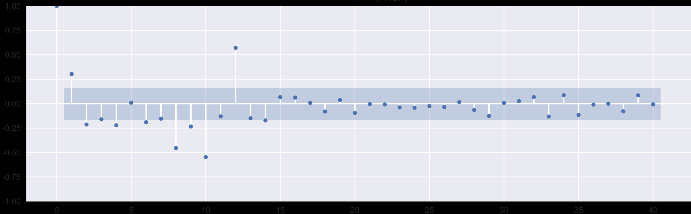
□□□□□□□□(PACF)
