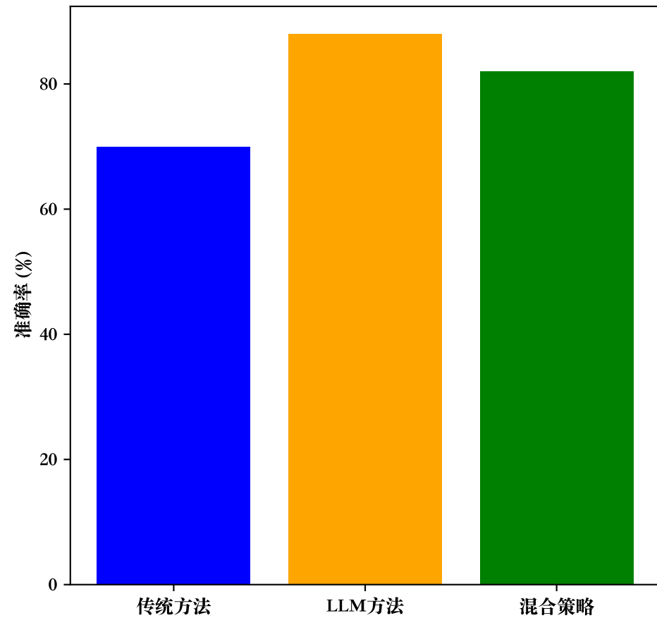
准确率比较
