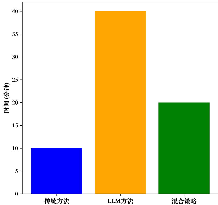
时间比较
