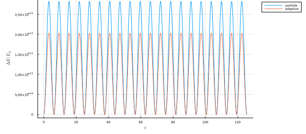
(d) Yoshida with fixed and adaptive timesteps
