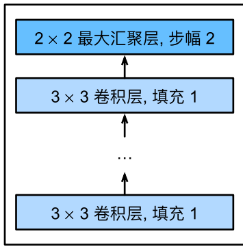
VGG 块
