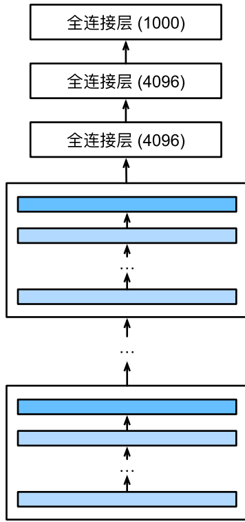
VGG
