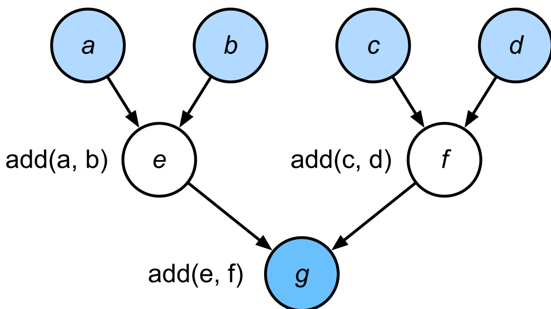
图 12.1.1 命令式编程中的数据流
