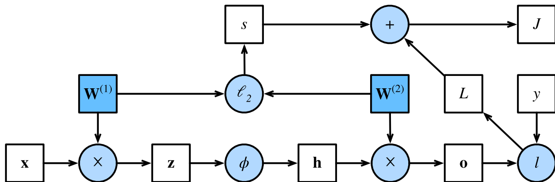
图 4.7.1 前向传播的计算图
