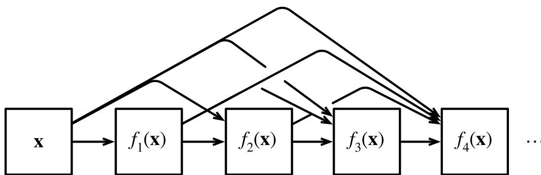
图 7.7.2 稠密连接。
