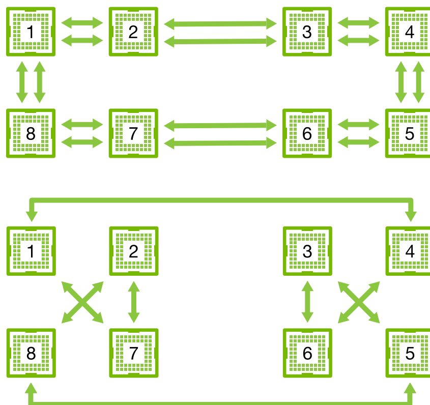
图 12.7.5 将 NVLink 网络分解为两个环。
