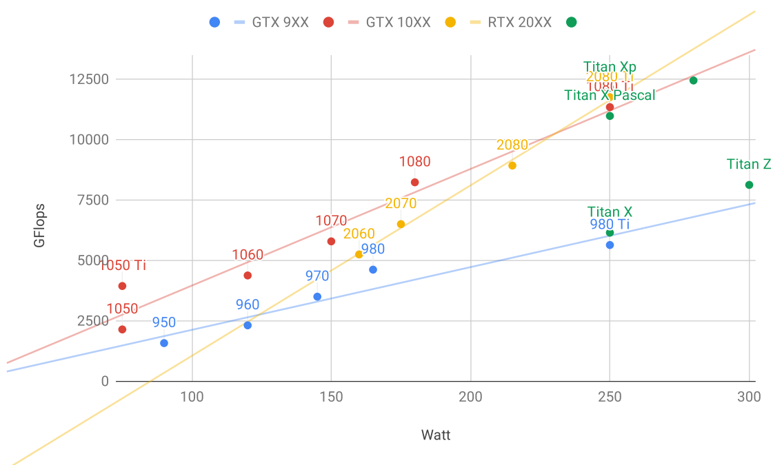
图 A.4.2 浮点计算能力和能耗
