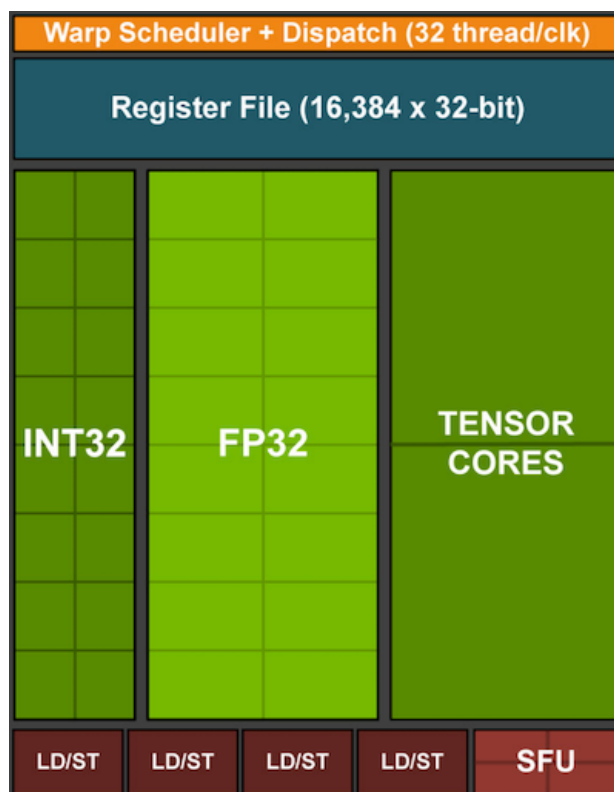
图 12.4.7 NVIDIA Turing 处理块（图片由英伟达提供）
