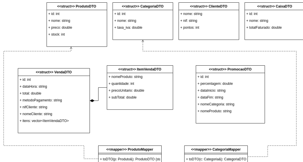
Fig. 9. Diagrama de DTOs e Mappers
