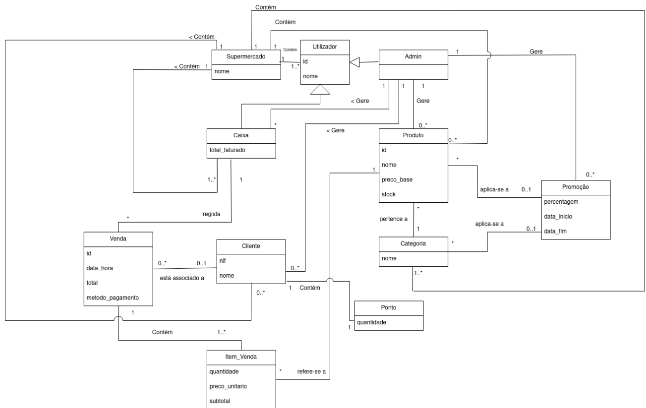
Fig. 1. Diagrama UML de Domínio
