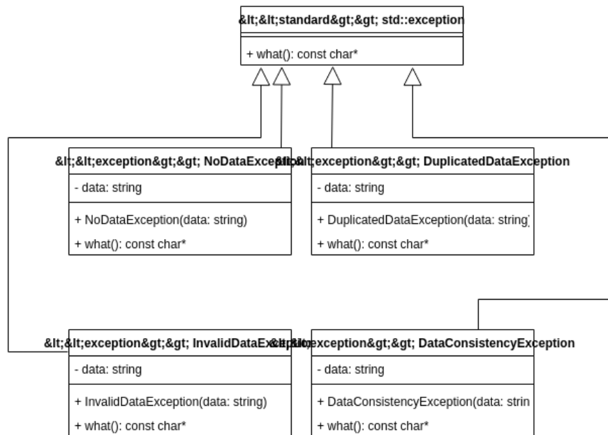
Fig. 6. Diagrama de Classes das Exceções
